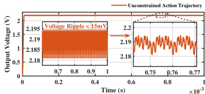
(d) Output Voltage Curve
