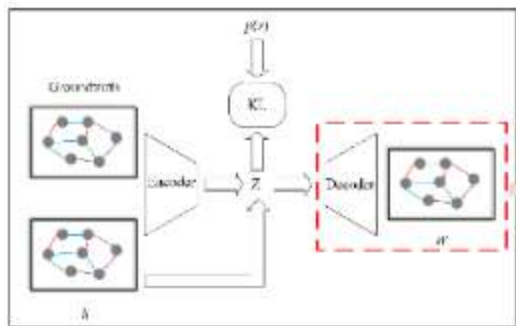
IDVAE
