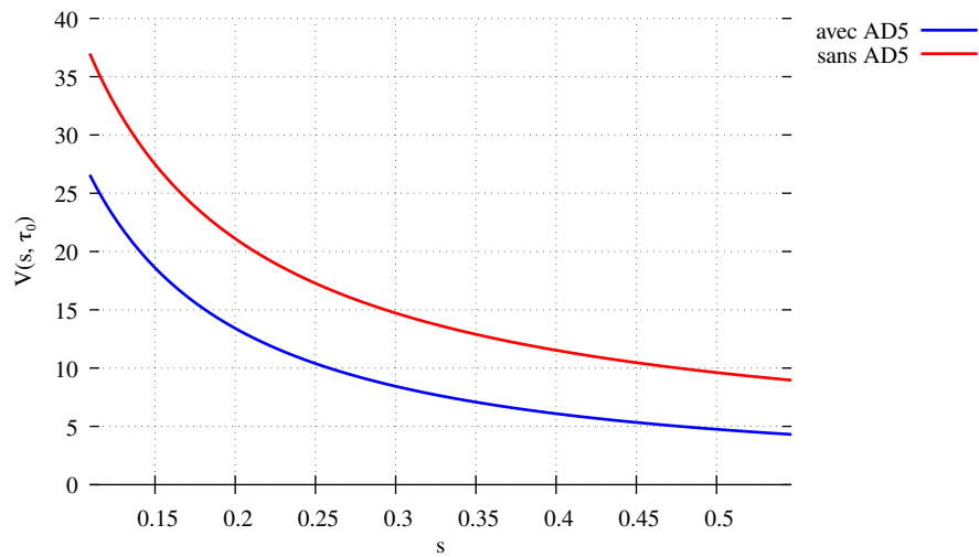
V(s) avec s = 0.2187
