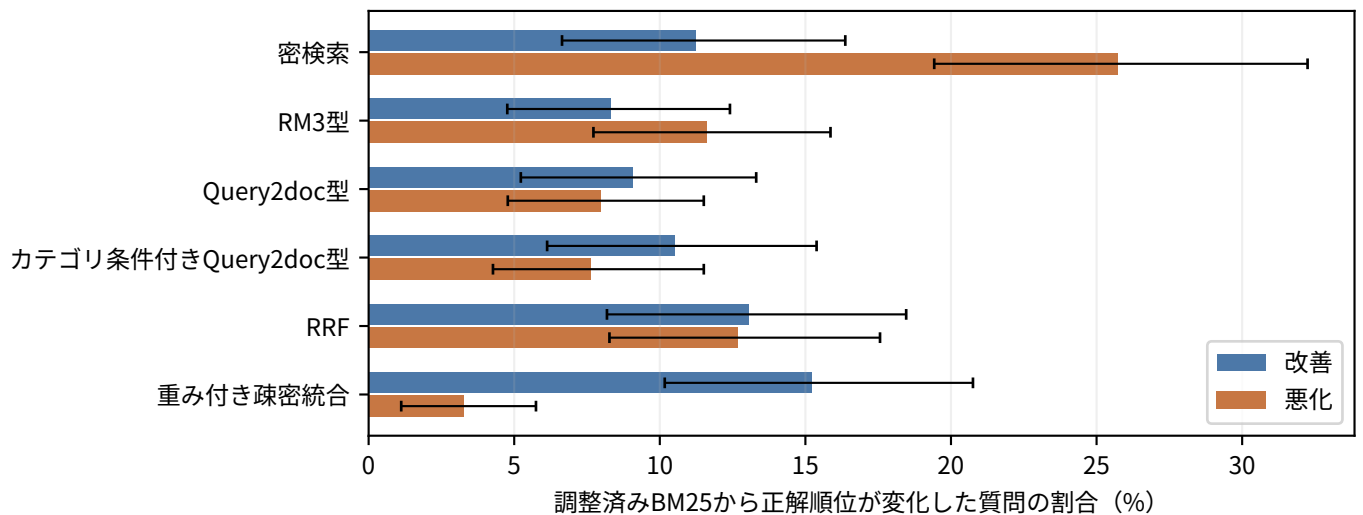
図2 調整済み BM25 に対する正解順位の改善・悪化率。順位不変は省略した。カテゴリ条件付き Query2doc 型は正解カテゴリを利用する。誤差棒は根拠文書単位の 95% クラスタ・ブートストラップ区間（多重比較未調整）。
