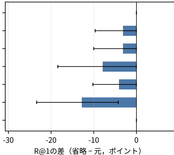
BM25
