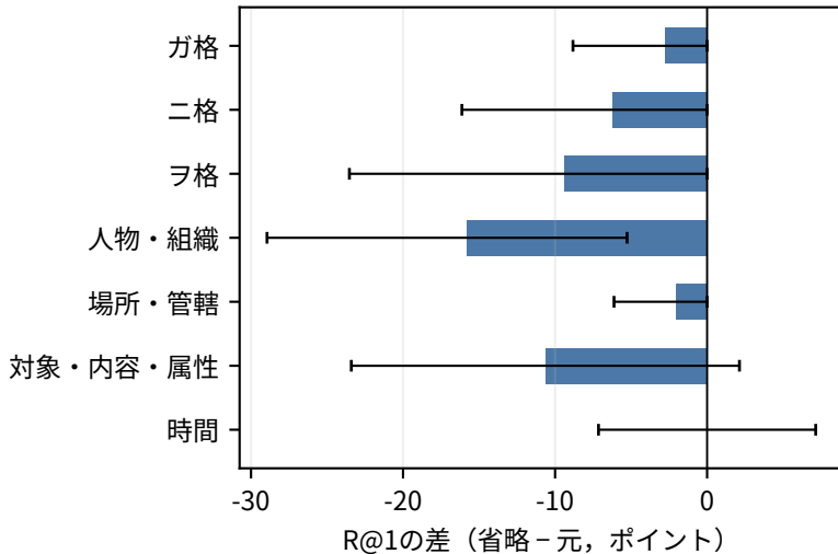
密検索
