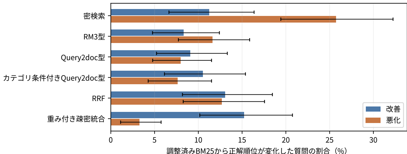
図2 調整済み BM25 に対する正解順位の改善・悪化率。順位不変は省略した。カテゴリ条件付き Query2doc 型は正解カテゴリを利用する。誤差棒は根拠文書単位の 95% クラスター・ブートストラップ区間（多重比較未調整）。
