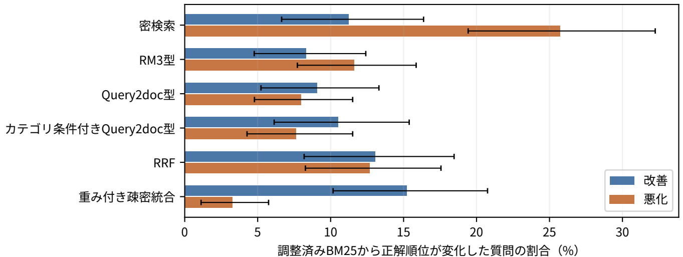
図2 調整済みBM25に対する正解順位の改善・悪化率。順位不変は省略した。カテゴリ条件付きQuery2doc型は正解カテゴリを利用する。誤差棒は根拠文書単位の95%クラスターブートストラップ区間（多重比較未調整）。
