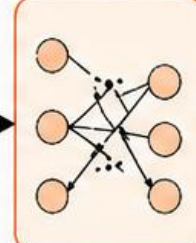
下游任务头
