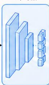
解码器
