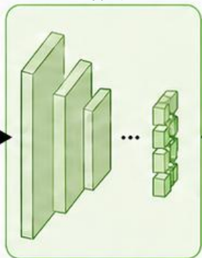
粗粒度编码
