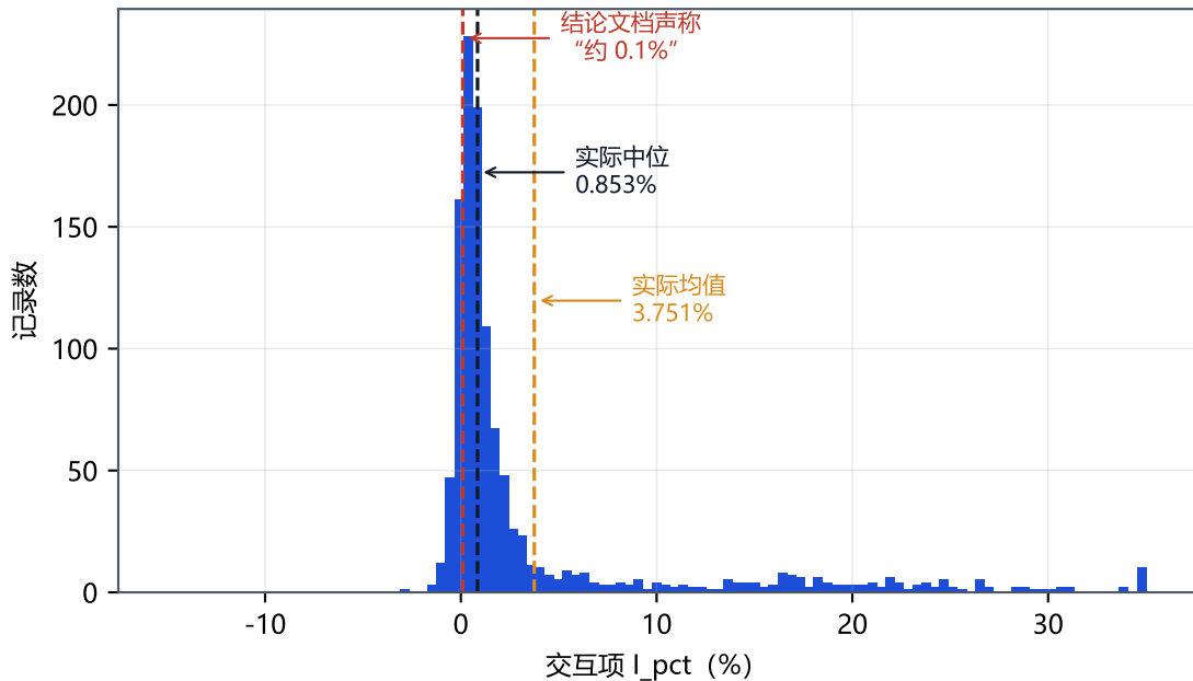
图 A8 交互项：绝对值 P95 达 21.69%、最大 65.94%， “交互很小、二乘二分解足够稳定” 不成立
