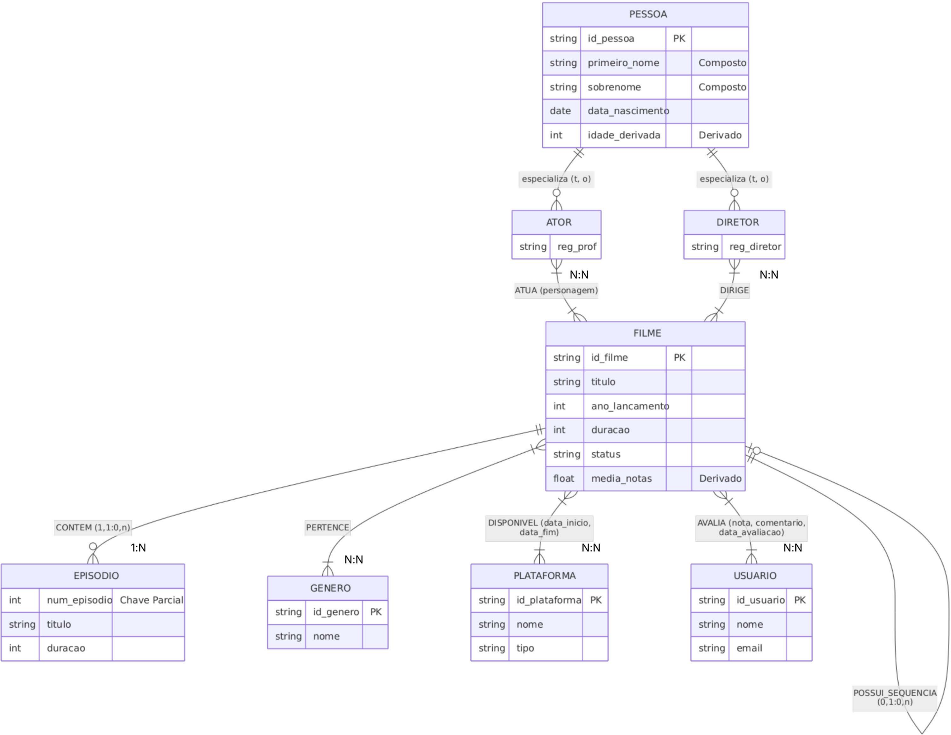
Diagrama ER - Cadastro de filmes
