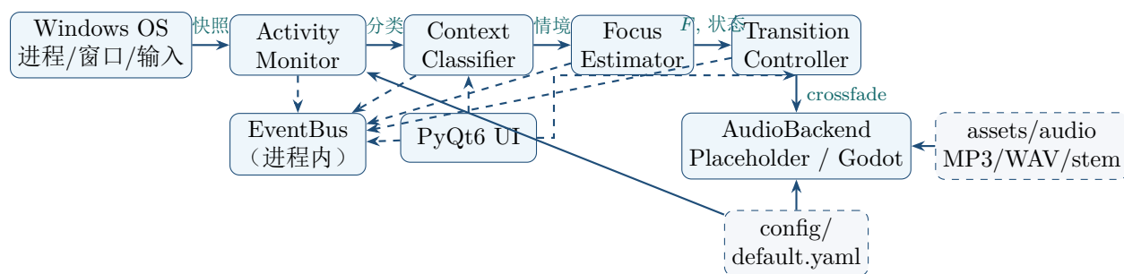
图 2: 系统模块依赖与数据流 (实线为主路径, 虚线为事件总线与 UI 干预)
