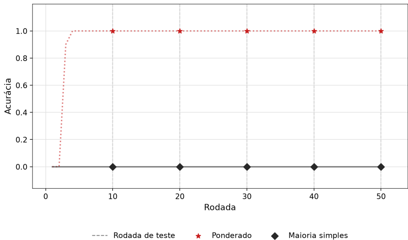
Figura 3. Consenso ponderado e maioria simples, 65% de nós maliciosos em conluio, 20 nós, EMA.
