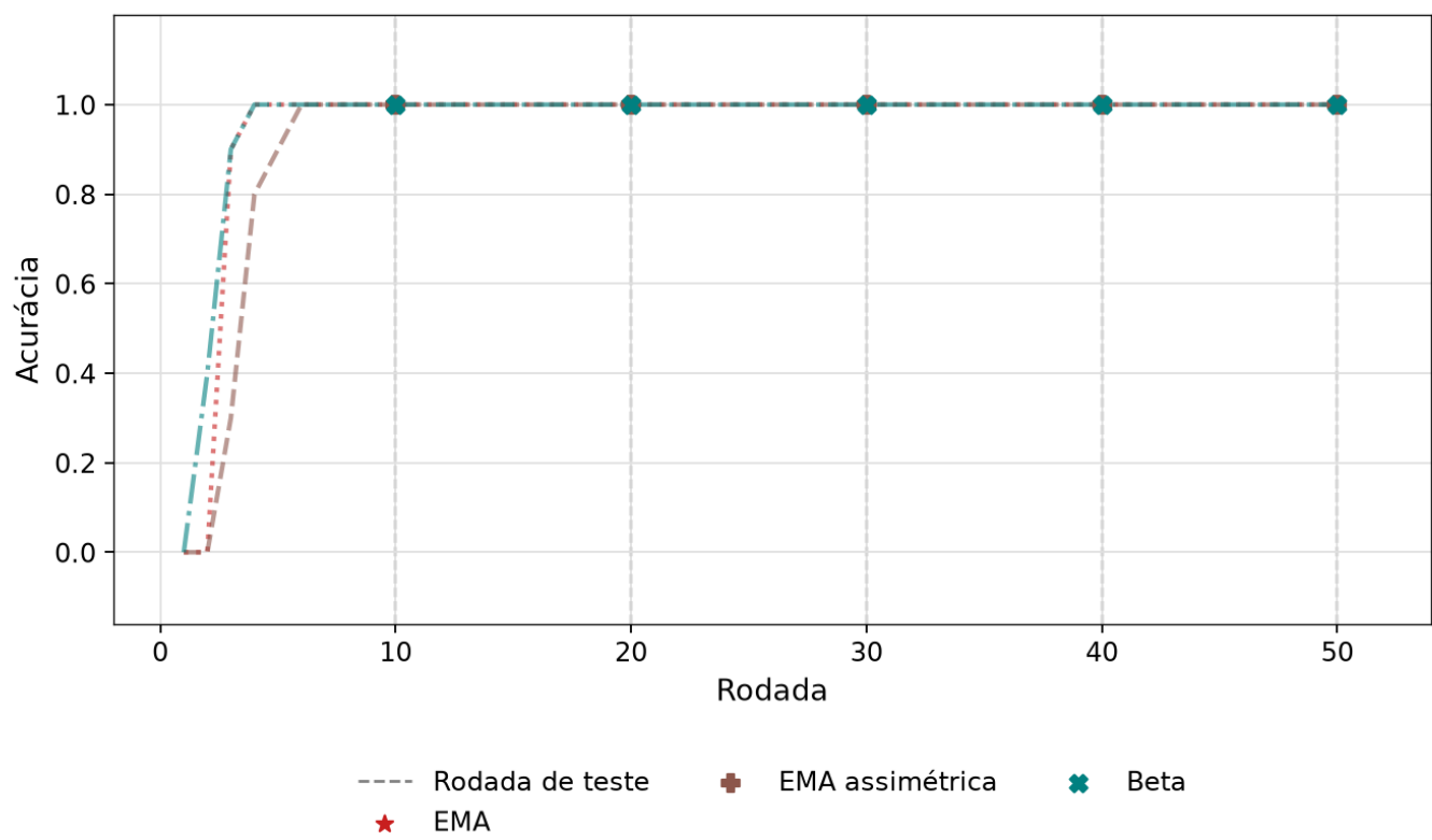
Figura 5. Acurácia do consenso ponderado por mecanismo, 65% em conluio, 20 nós. EMA, EMA assimétrica e Beta chegam a 1,000 antes da rodada 10 e permanecem nesse valor nos testes.
