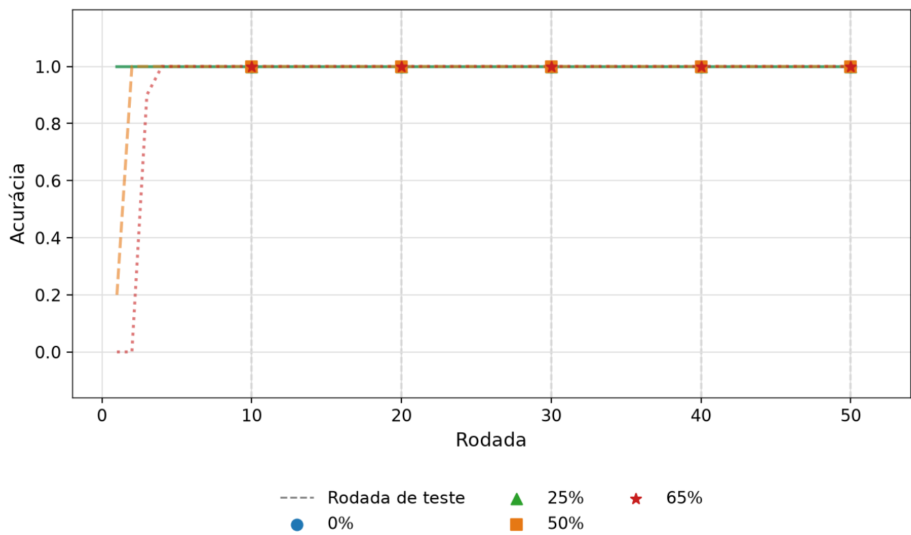
Figura 1. Acurácia do consenso ponderado por rodada, com conluio, 20 nós, EMA. A curva de 0% é o cenário sem maliciosos. A série de 65% é a linha vermelha pontilhada com estrela.
