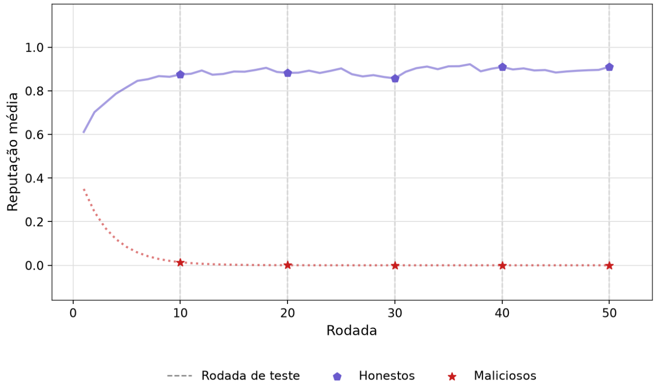
Figura 4. Reputação média dos honestos e dos maliciosos, 65% em conluio, 20 nós, EMA. A reputação dos maliciosos é a linha vermelha pontilhada com estrela.
