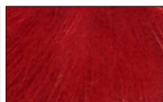
8017 RED SKY
