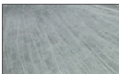
8019 RAIN CLOUD
