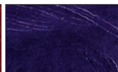
8018 MONSOON MAUVE
