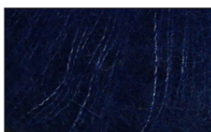
8016 NAVY NIGHT
