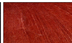
8012 ORANGE PEEL
