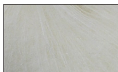
8001 ICICLE
