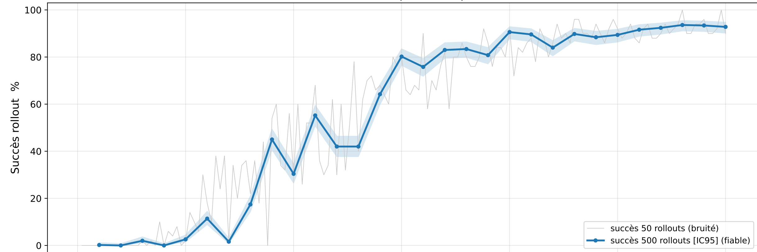
Can ResNet34 birdview — succès par checkpoint (50 vs 500 rollouts)
