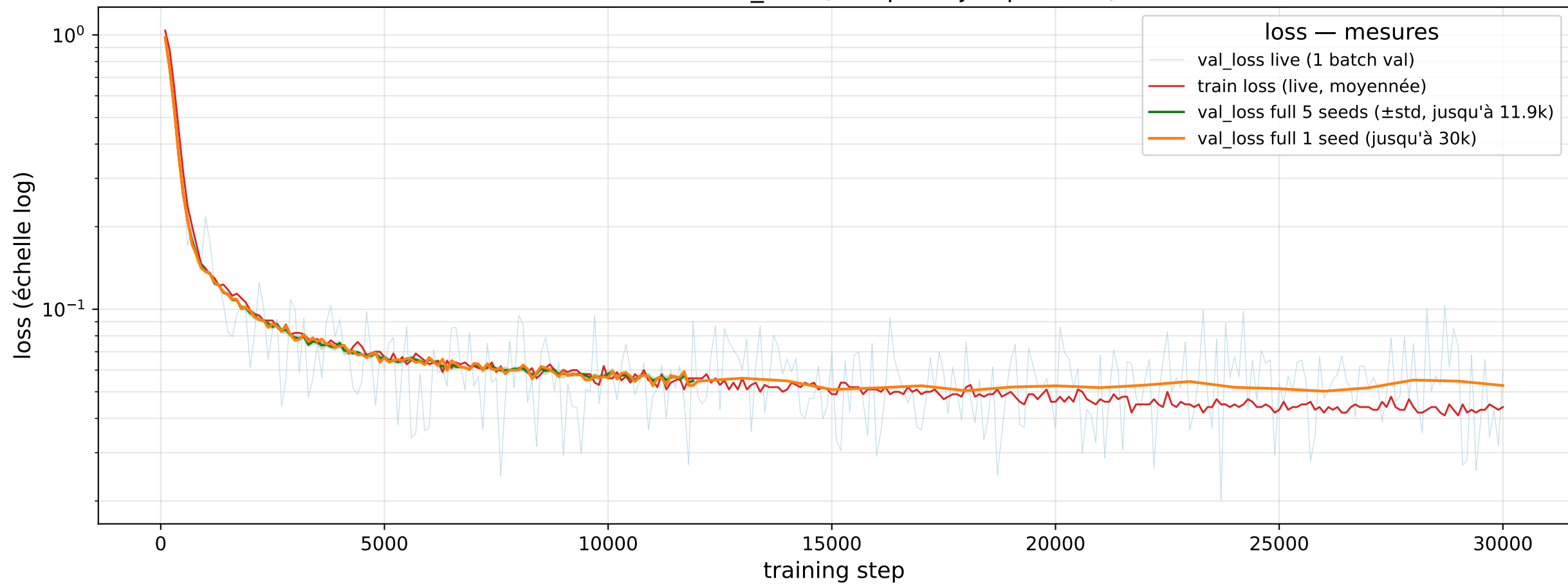
train loss vs val_loss (complète jusqu'à 30k)
