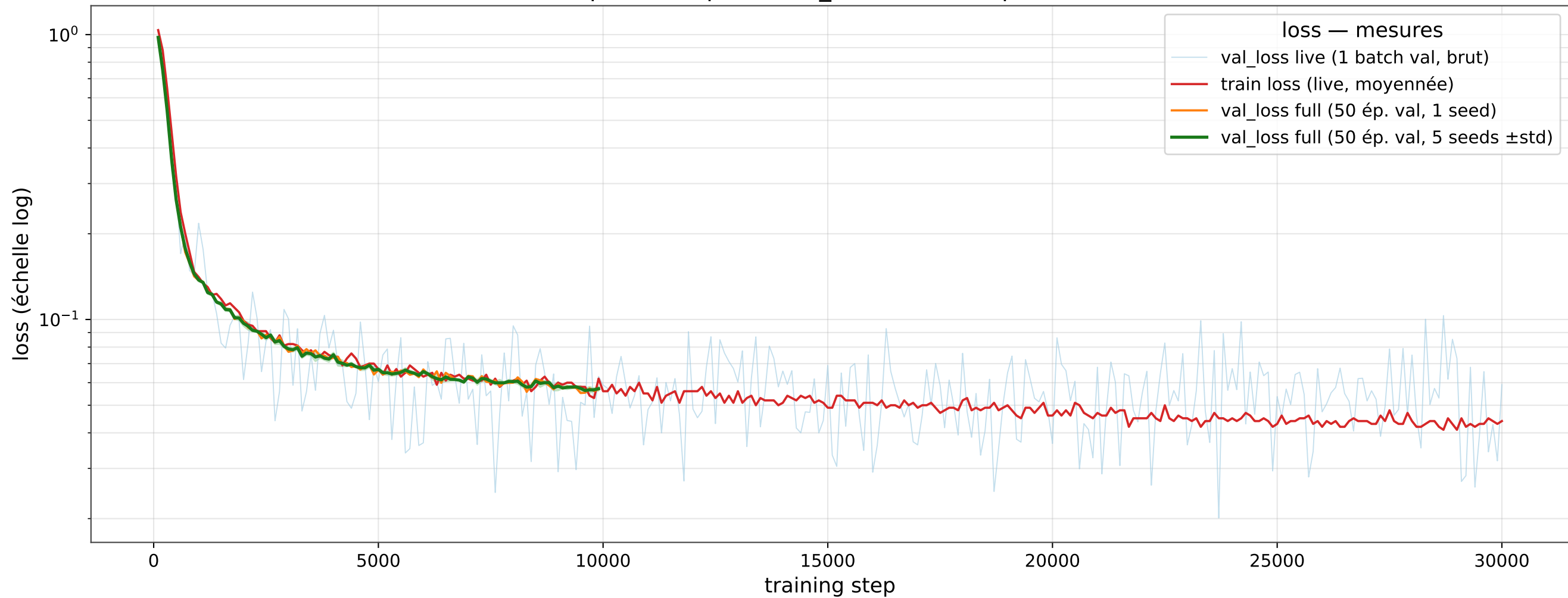
Toutes les loss par checkpoint (val_loss full -&gt; step 9900, 05 en cours)
