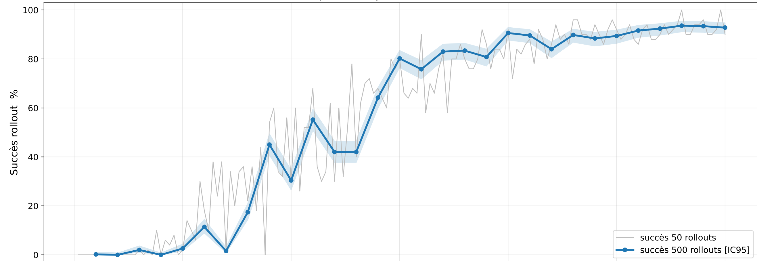
Succès par checkpoint — 50 vs 500 rollouts
