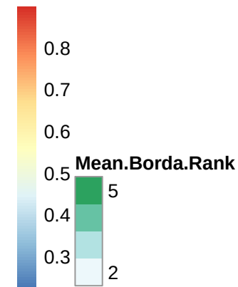
C-Index
