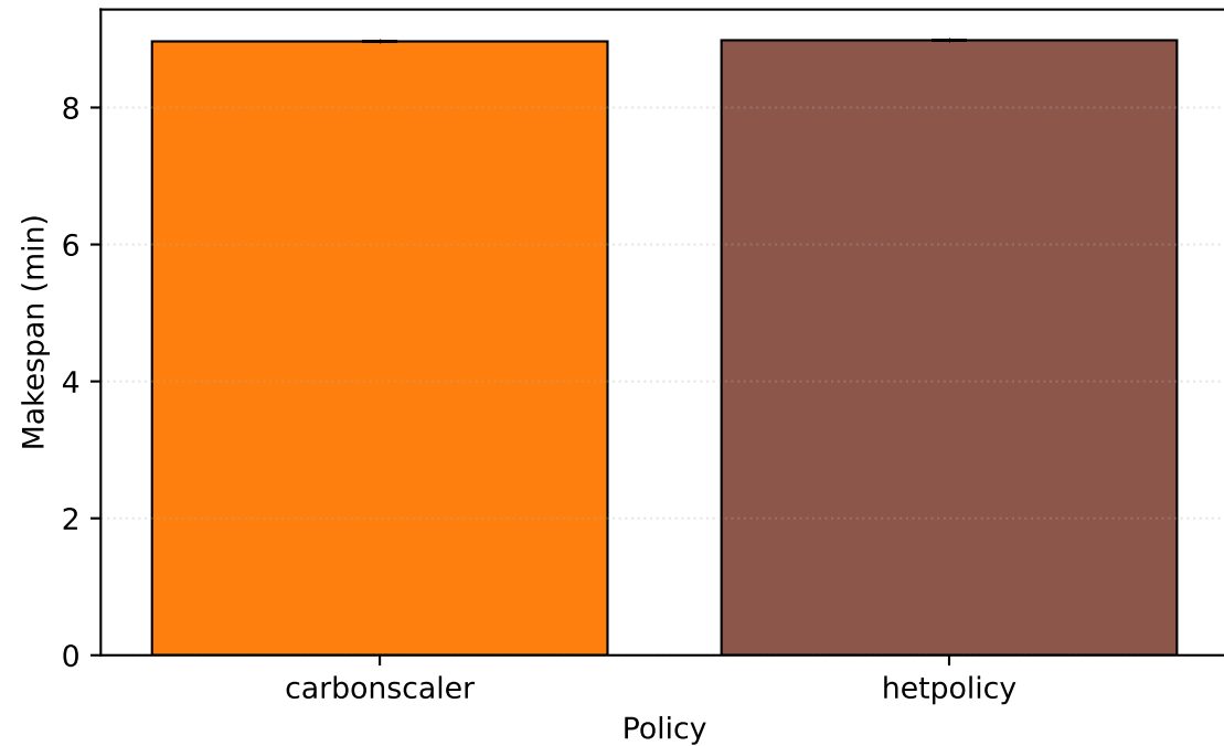
K8S makespan (median \pm 95% CI)
