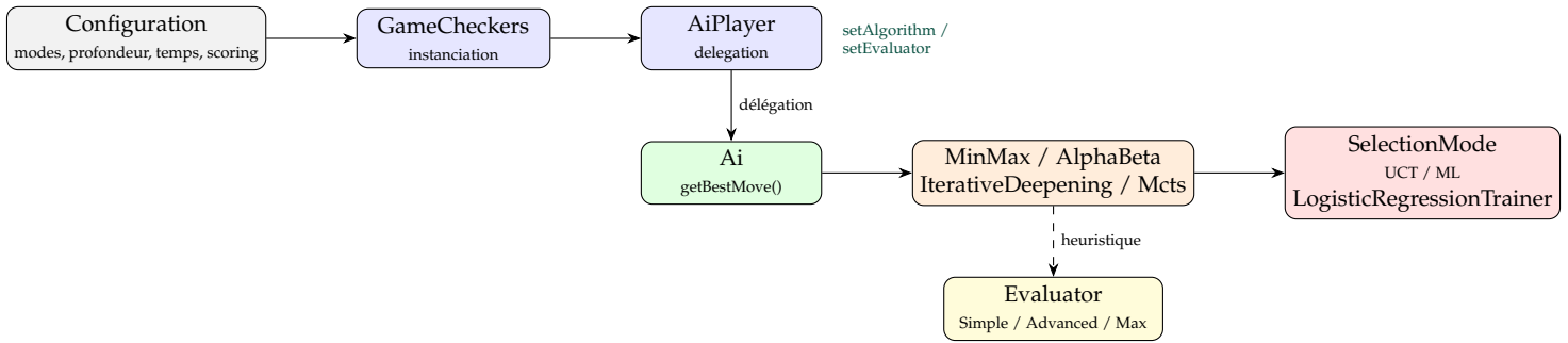
FIGURE 22 – Chaîne de dépendance du module Intelligence Artificielle
