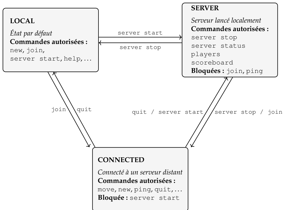
FIGURE 23 – Modes d’exécution du client et commandes autorisées selon ClientMode .
