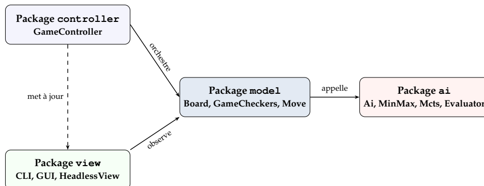
FIGURE 15 – Diagramme de packages simplifié (vue d'ensemble MVC + IA)
