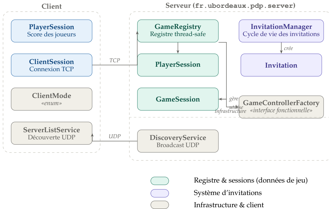
FIGURE 21 – Architecture structurelle de la couche réseau
