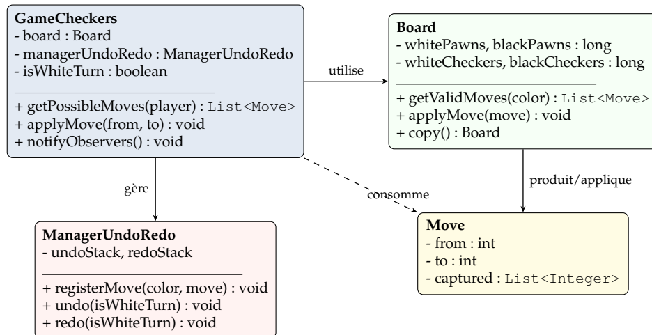
FIGURE 16 – Diagramme de classes UML simplifié du moteur de jeu
