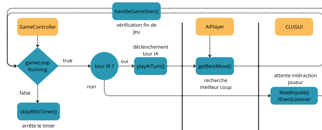
FIGURE 18 – Boucle de contrôle du jeu
