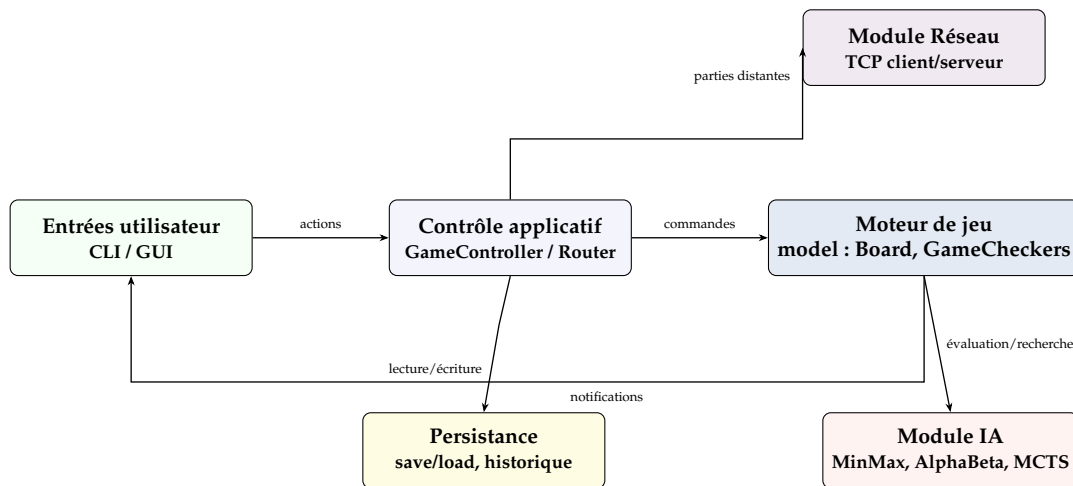
FIGURE 14 – Diagramme simplifié de l'architecture globale du projet
