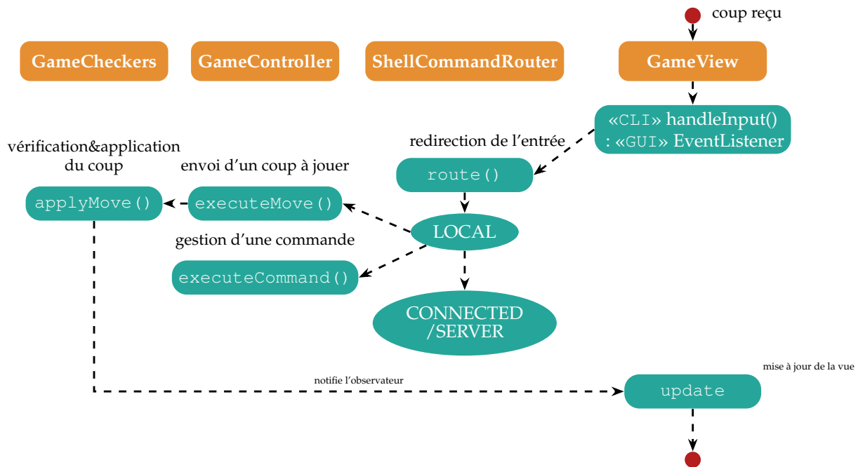
FIGURE 17 – Interaction entre le moteur et la vue via le contrôleur
