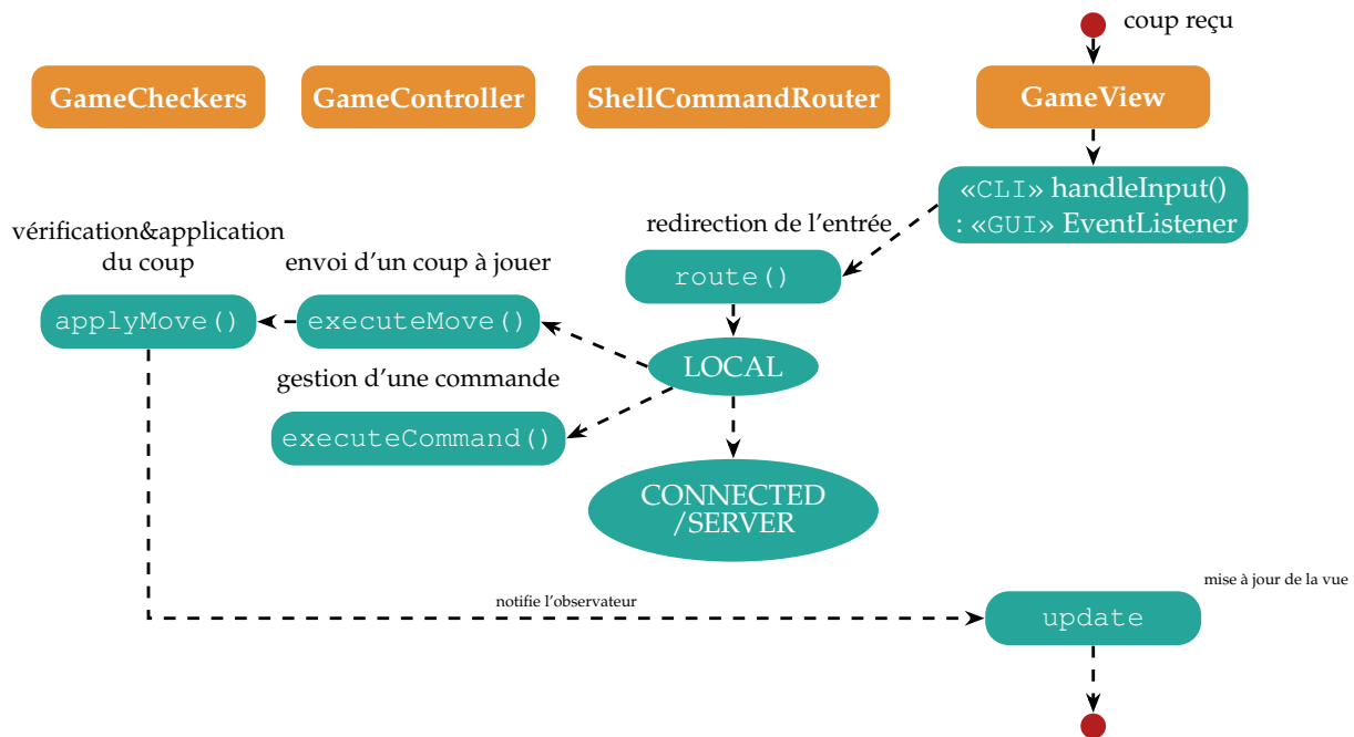
FIGURE 14 – Interaction entre le moteur et la vue via le contrôleur
