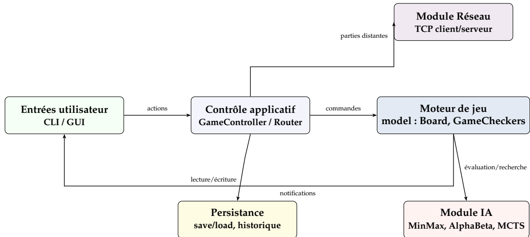
FIGURE 11 – Diagramme simplifié de l’architecture globale du projet
