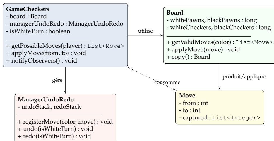
FIGURE 13 – Diagramme de classes UML simplifié du moteur de jeu
