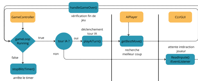
FIGURE 15 – Boucle de contrôle du jeu
