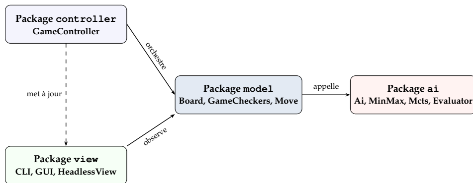
FIGURE 12 – Diagramme de packages simplifié (vue d’ensemble MVC + IA)
