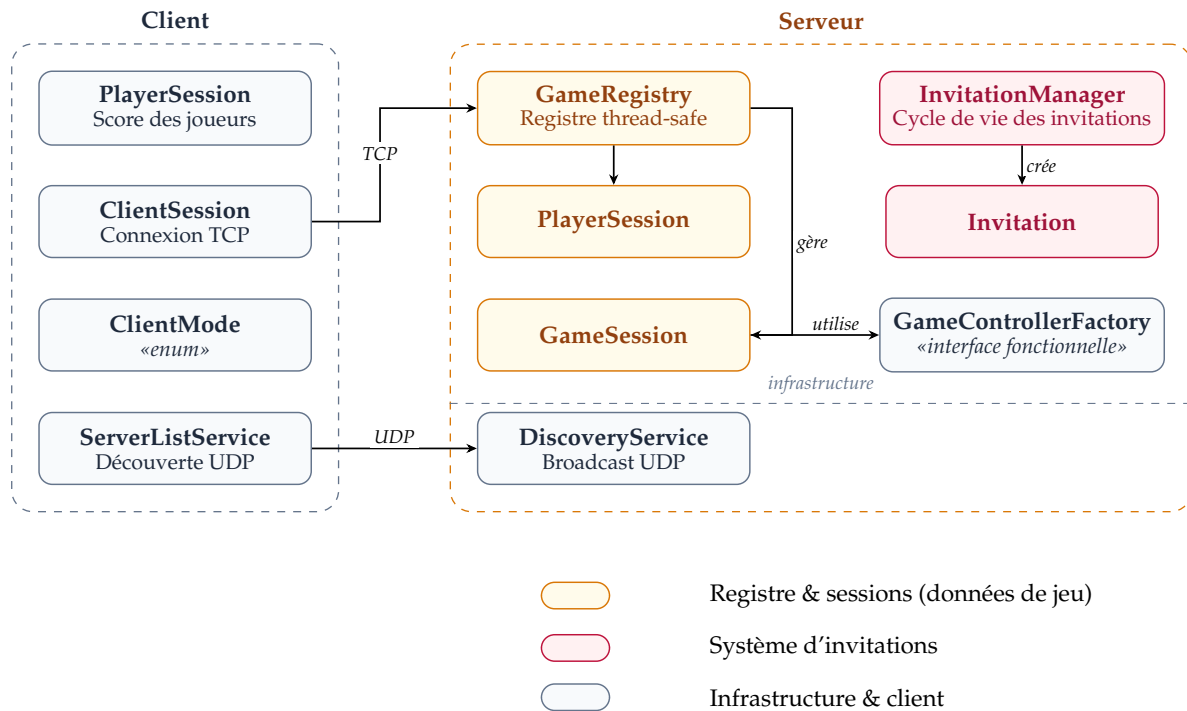
FIGURE 17 – Architecture structurelle de la couche réseau
