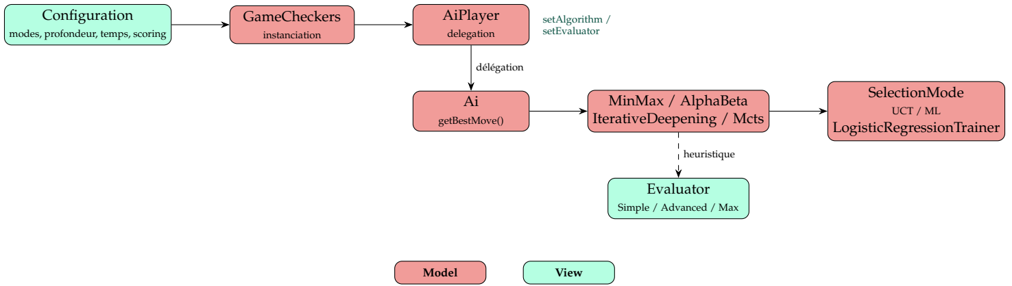
FIGURE 18 – Chaîne de dépendance du module Intelligence Artificielle
