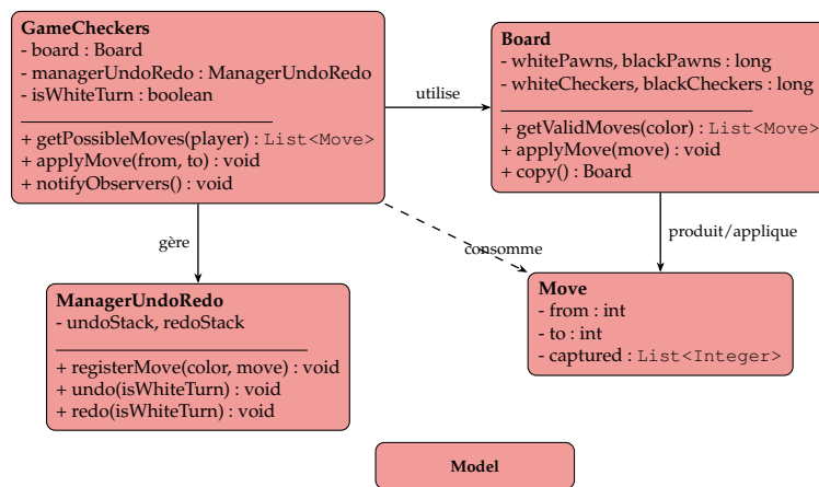
FIGURE 12 – Diagramme de classes UML simplifié du moteur de jeu
