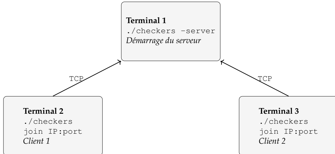
FIGURE 20 – Exemple minimal de lancement d'une partie en ligne : un serveur et deux clients sur trois terminaux distincts.
