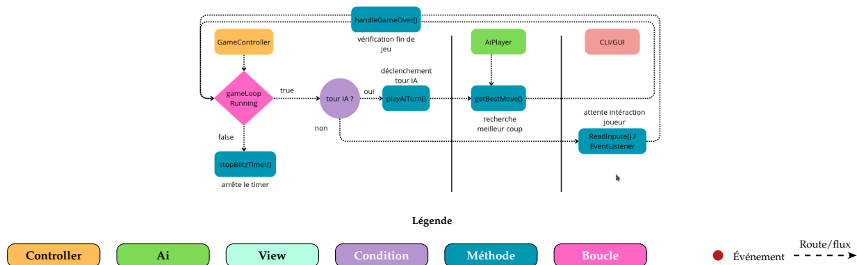
FIGURE 14 – Boucle de contrôle du jeu
