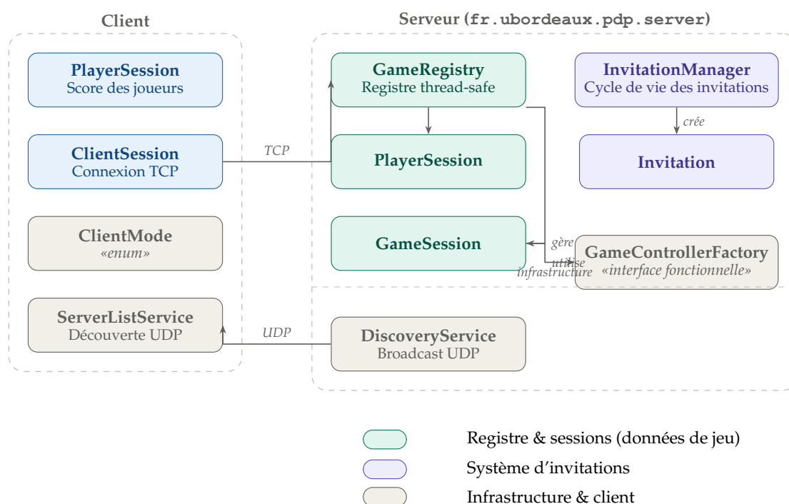
FIGURE 17 – Architecture structurelle de la couche réseau
