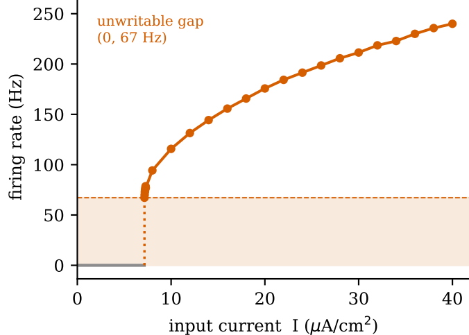
D Wang-Buzsaki interneuron (Type-I)
