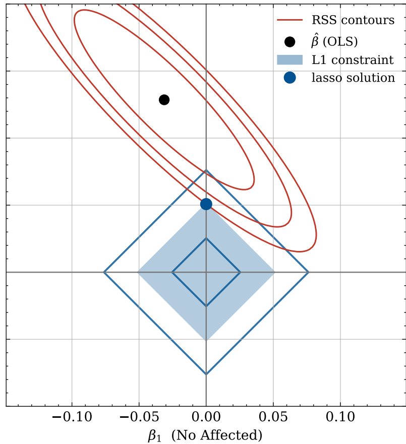
Lasso (L1)
