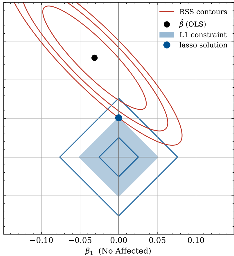
Lasso (L1)
