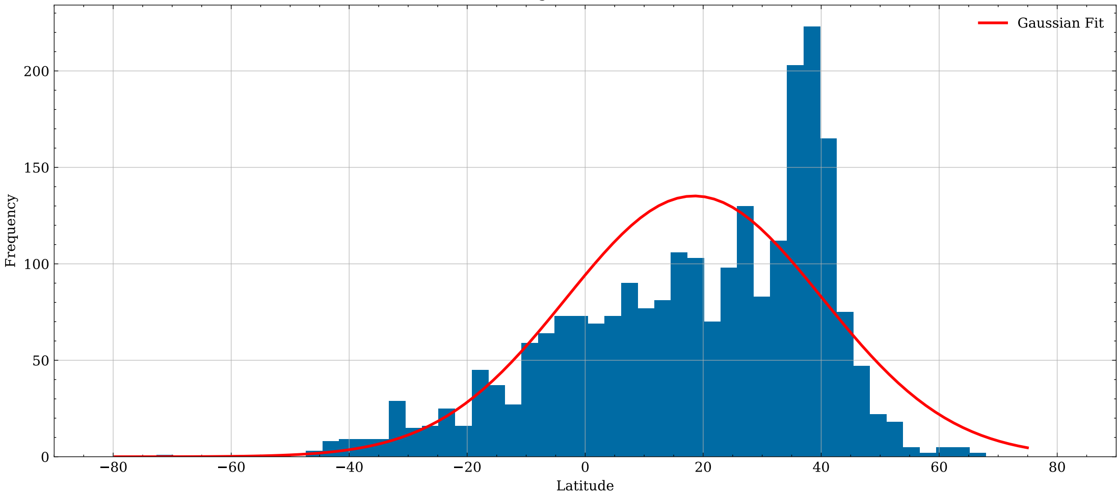
Histogram of Latitude
