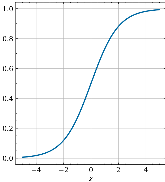
Sigmoid
