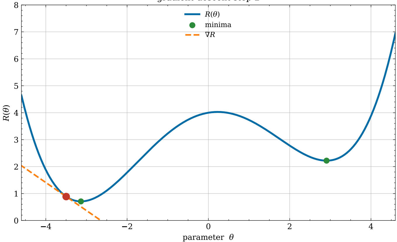
gradient-descent step 2
