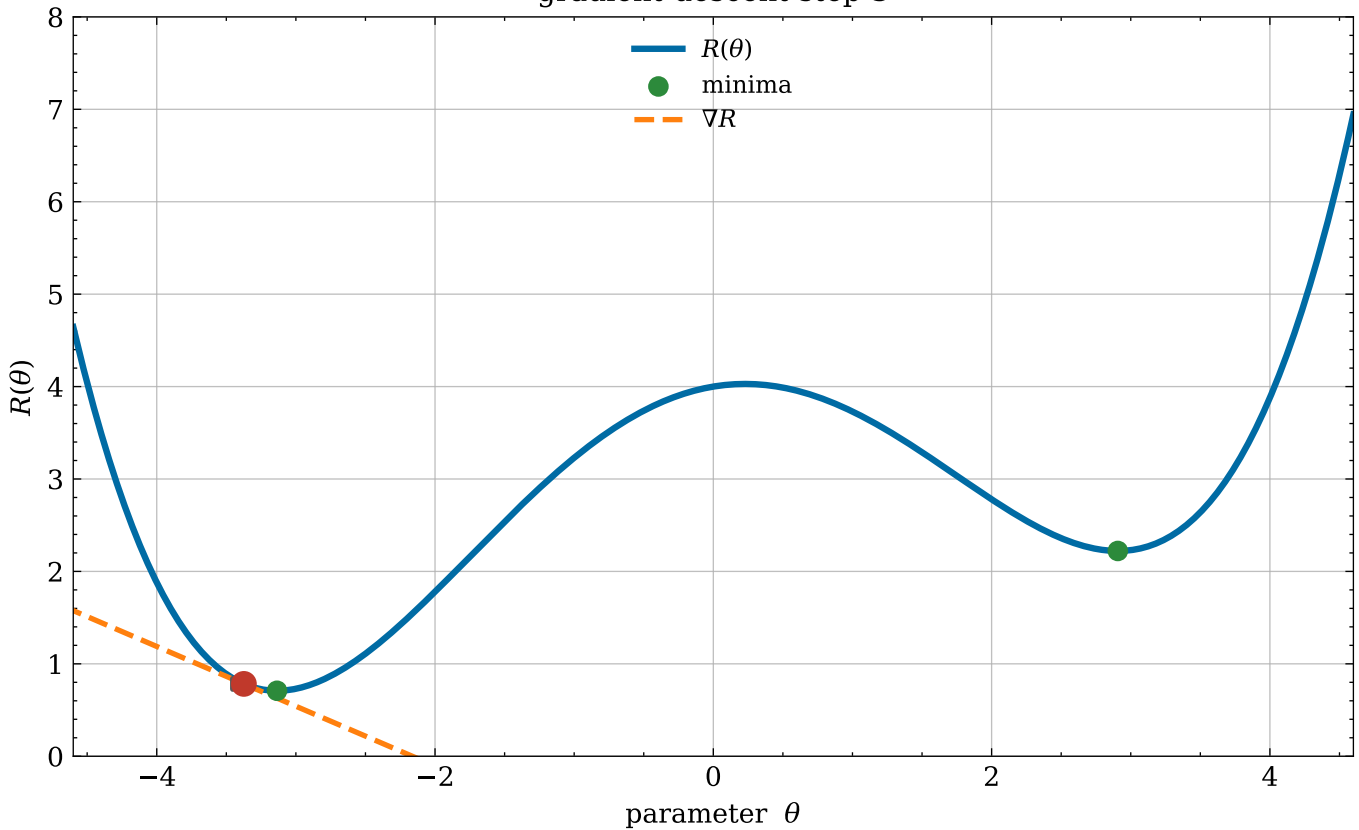
gradient-descent step 3
