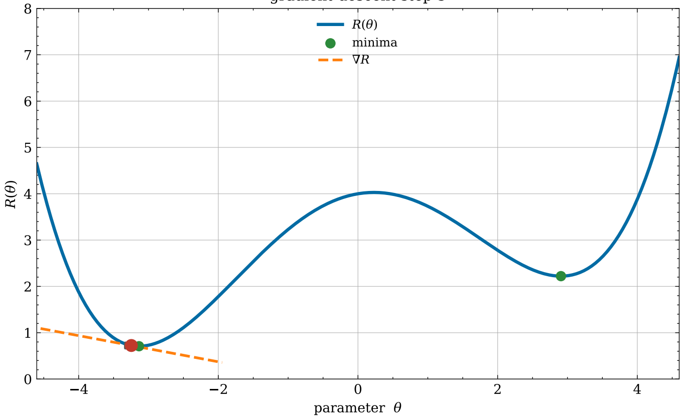
gradient-descent step 5
