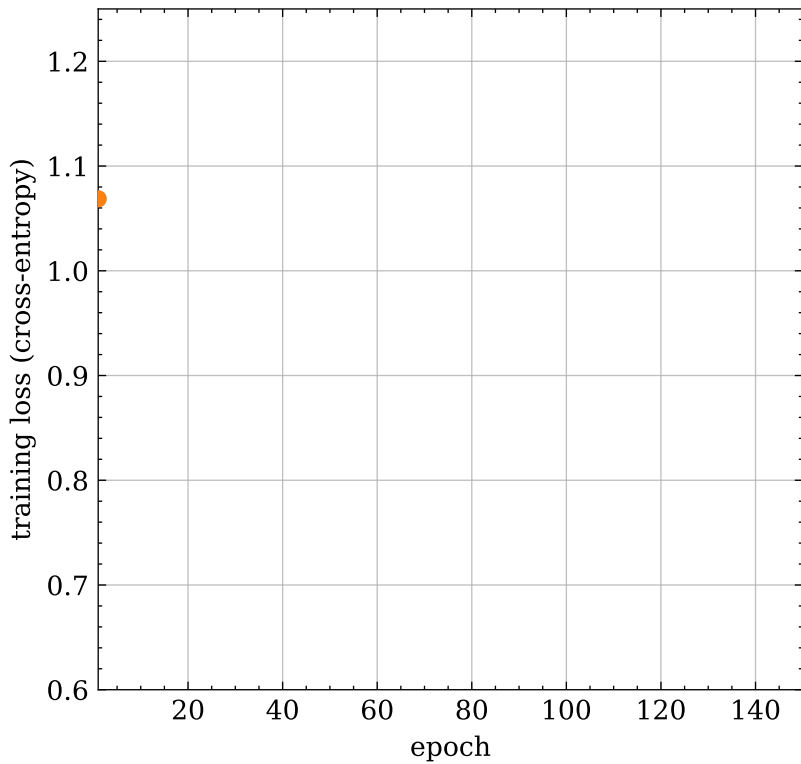
epoch 1
