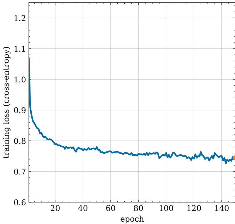
epoch 150
