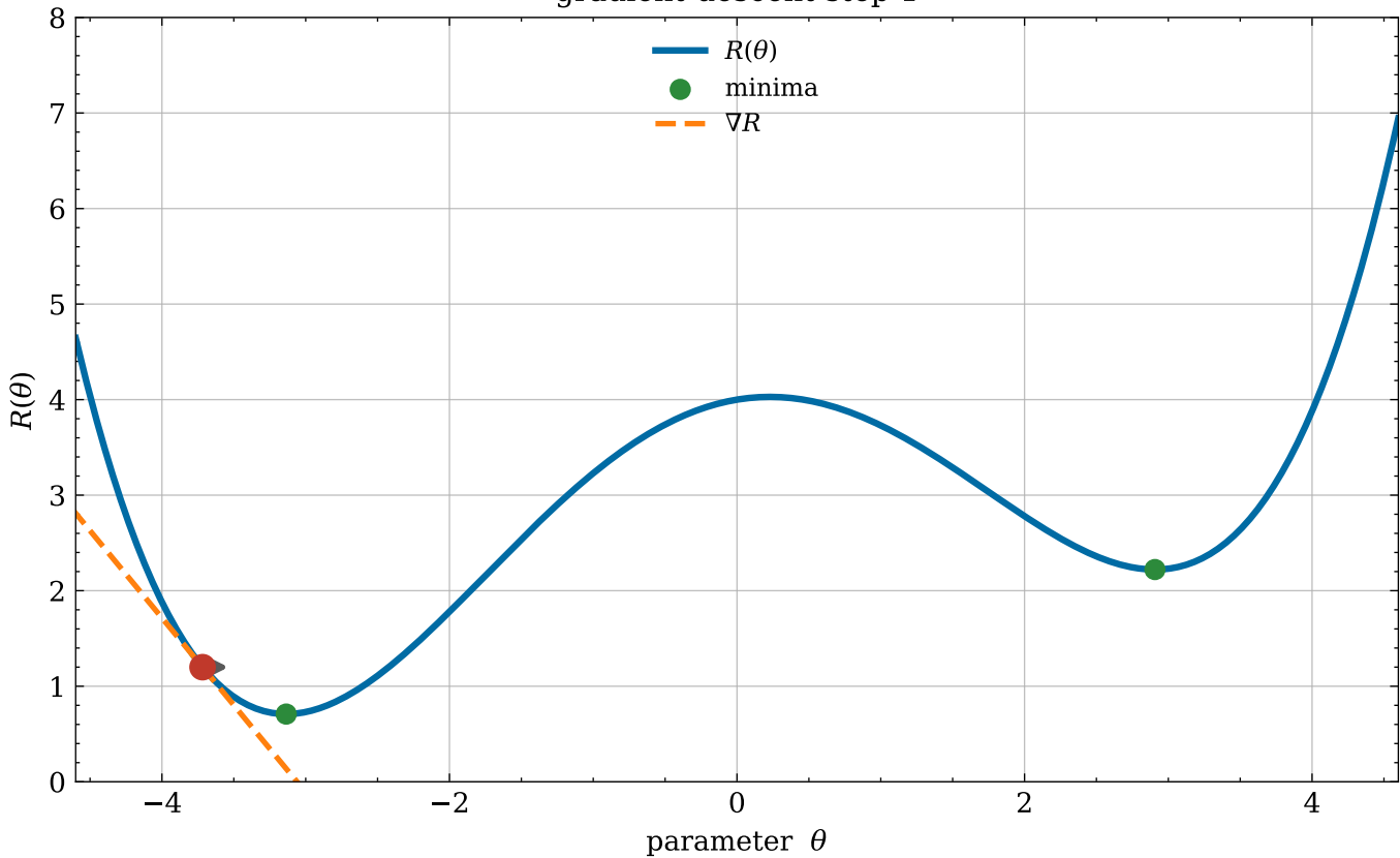
gradient-descent step 1
