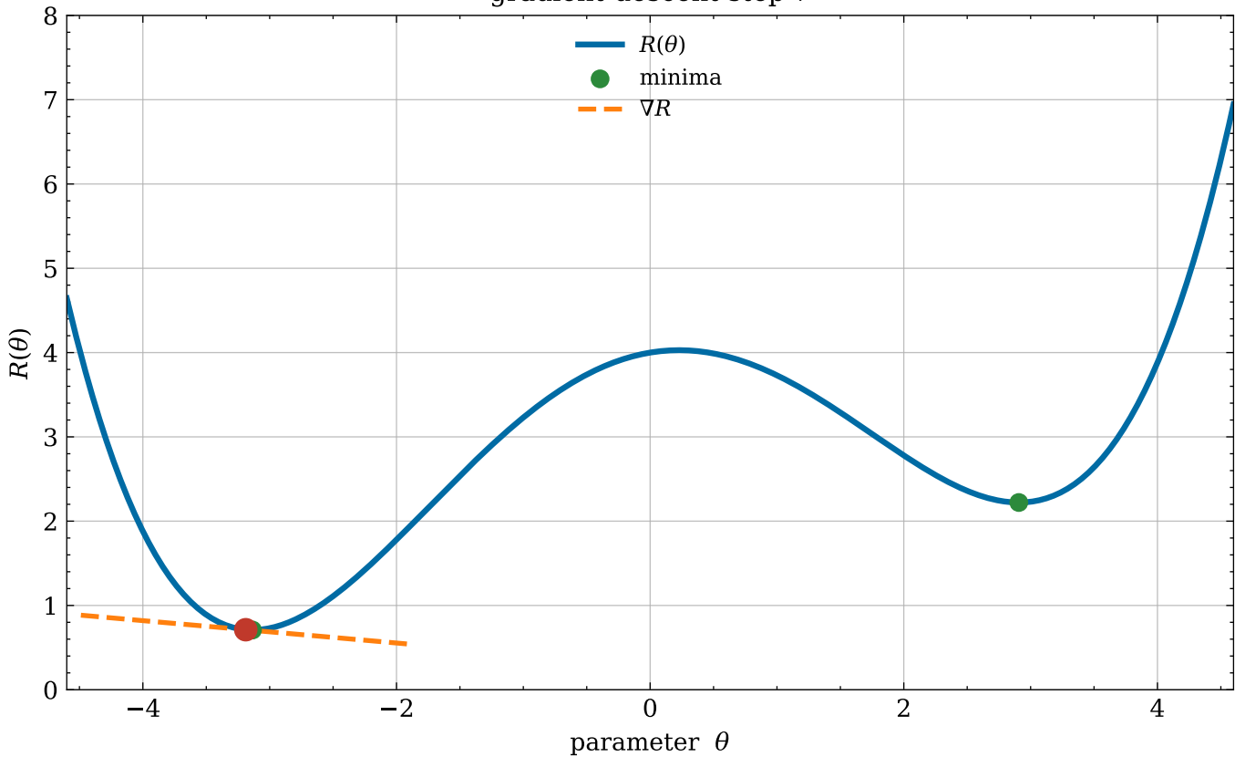
gradient-descent step 7
