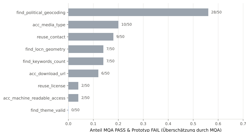
Abbildung 6.9: Überschätzungsrate je Klasse-B-Indikator: Anteil MQA PASS & Prototyp FAIL (Kernstichprobe)
