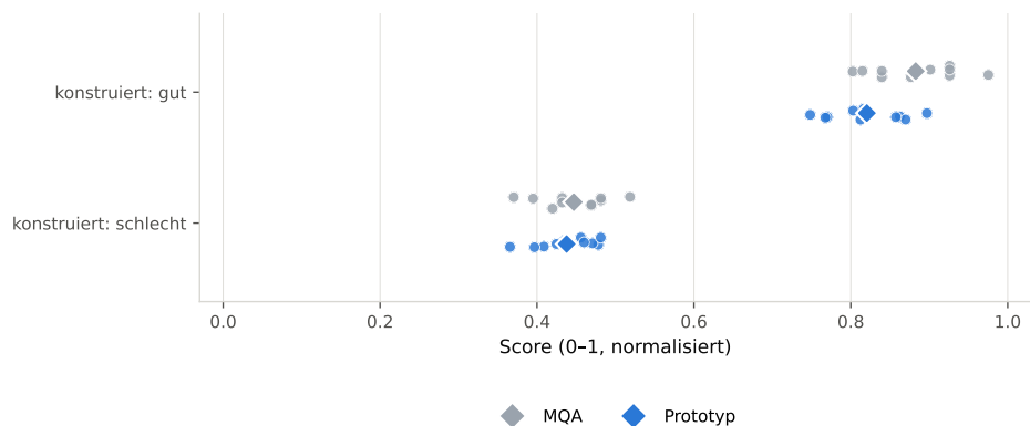
Abbildung 6.14: Score-Trennschärfe von MQA und Prototyp nach Konstruktionsabsicht (Extremfälle, n = 20 , normalisierte 0–1-Skala)
