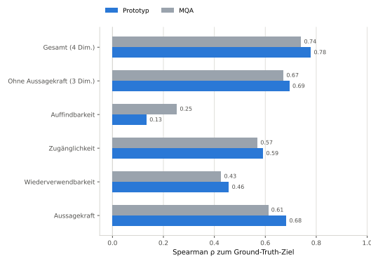
Abbildung 6.12: Triangulation gegen die Ground Truth: Spearman \rho von Prototyp und MQA je Zieldimension (Kernstichprobe, n = 50 )
