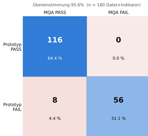
Abbildung K.1: Konvergenz auf Klasse-A-Indikatoren (Extremfälle, n = 180 Datei-Indikator-Paare)
