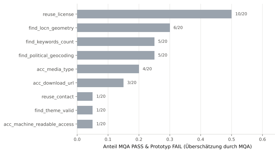
Abbildung K.2: Überschätzungsrate je Klasse-B-Indikator: Anteil MQA PASS & Prototyp FAIL (Extremfälle)
