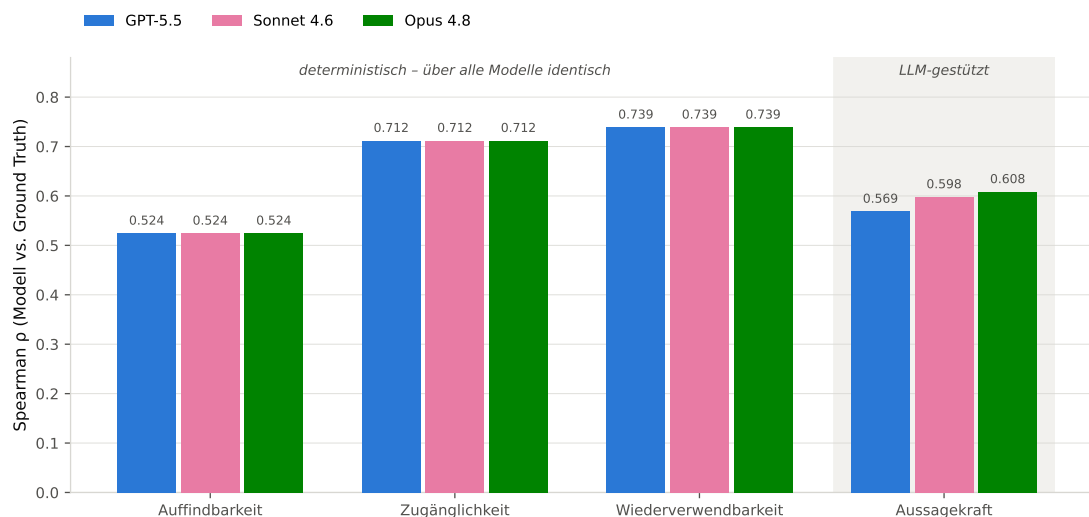
Abbildung 6.1: Spearman-Rangkorrelation zur Ground Truth je Qualitätsdimension und Sprachmodell (Kernstichprobe, n = 50 )
