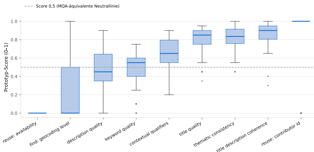
Abbildung 6.10: Prototyp-Score-Verteilung auf Klasse-C-Indikatoren, für die die MQA keine Metrik besitzt (Kernstichprobe)
