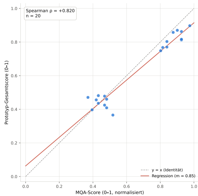
Abbildung K.4: Gesamtscore Prototyp vs. MQA (Extremfälle, n = 20 )
