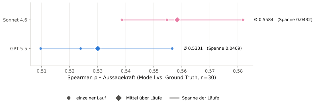
Abbildung 6.2: Spearman \rho der Aussagekraft über je drei Wiederholungsläufe, identische Teilstichprobe ( n = 30 )
