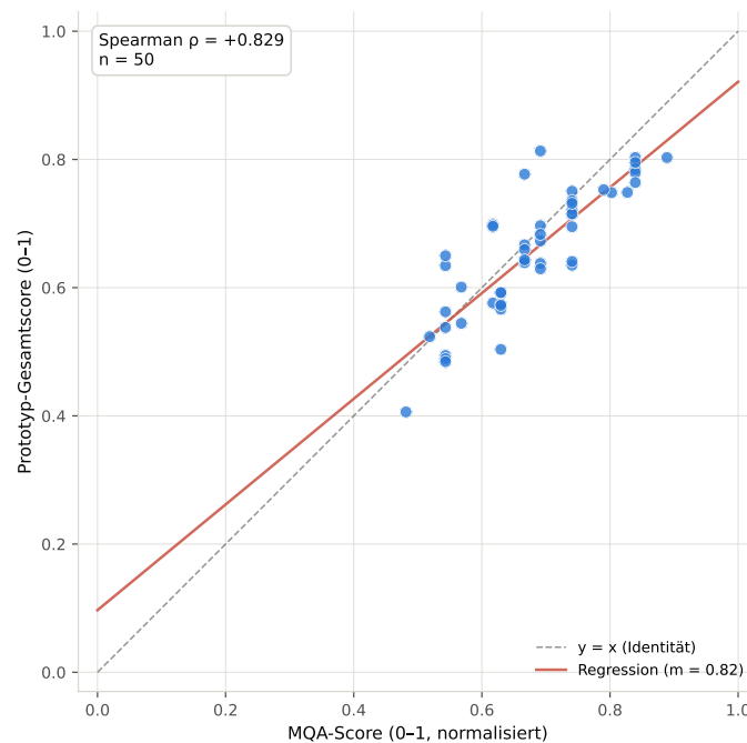
Abbildung 6.11: Gesamtscore Prototyp vs. MQA (Kernstichprobe, n = 50 )
