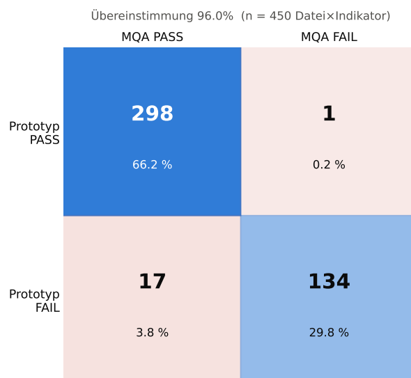
Abbildung 6.8: Konvergenz auf Klasse-A-Indikatoren (Kernstichprobe, n = 450 Datei-Indikator-Paare)
