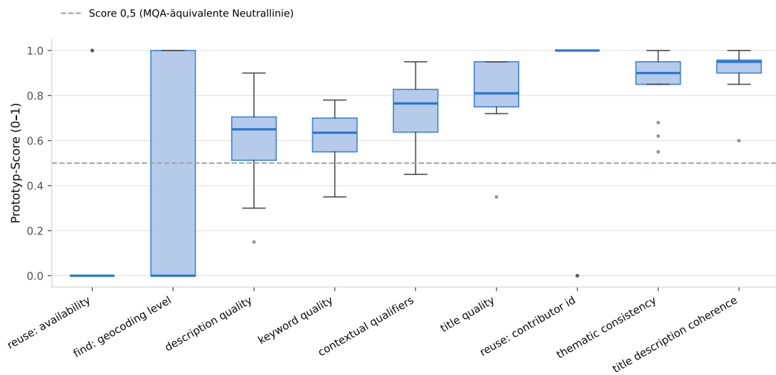
Abbildung K.3: Prototyp-Score-Verteilung auf Klasse-C-Indikatoren, für die die MQA keine Metrik besitzt (Extremfälle)
