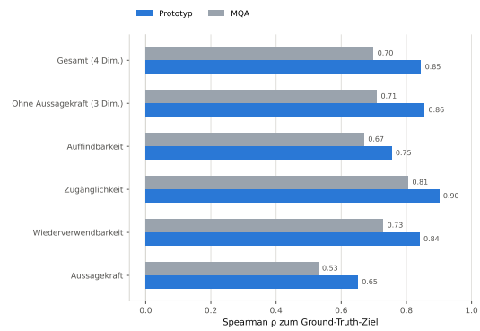
Abbildung 6.13: Triangulation gegen die Ground Truth: Spearman \rho von Prototyp und MQA je Zieldimension (Extremfälle, n = 20 )
