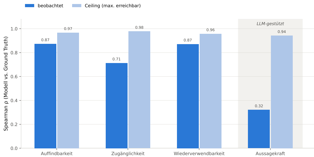
Abbildung 6.6: Spearman \rho je Qualitätsdimension, beobachtet vs. Ceiling (Extremfälle, n = 20 )
