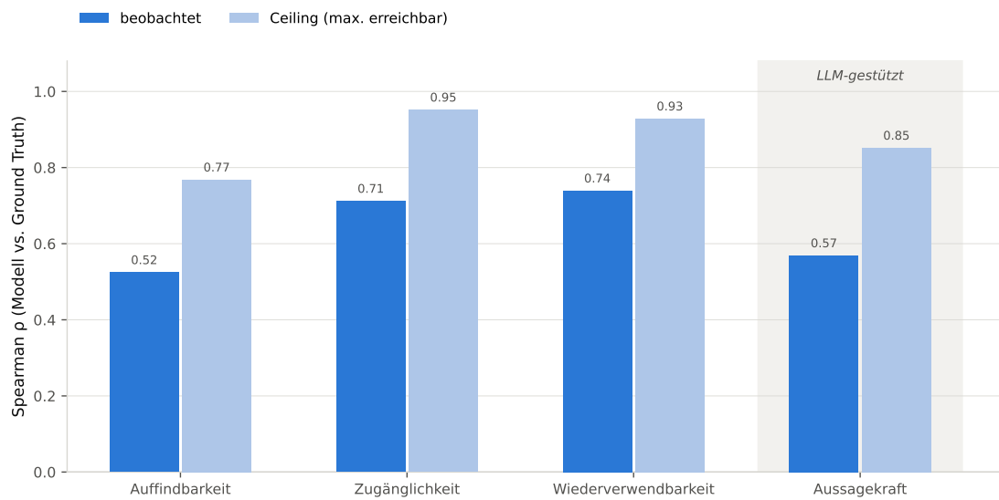
Abbildung 6.3: Spearman \rho je Qualitätsdimension, beobachtet vs. Ceiling (Kernstichprobe, n = 50 )
