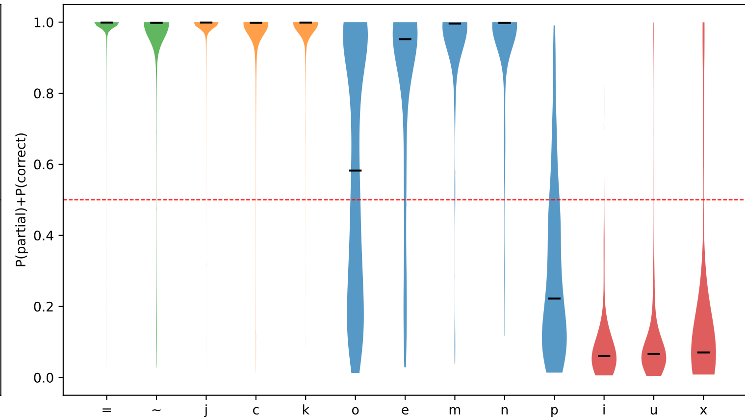
P(partial)+P(correct)
