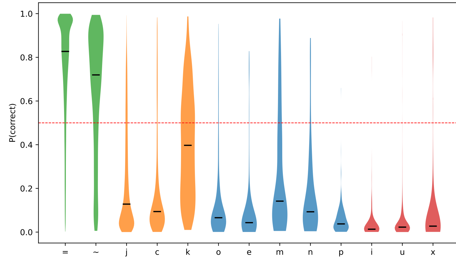
P(correct)
