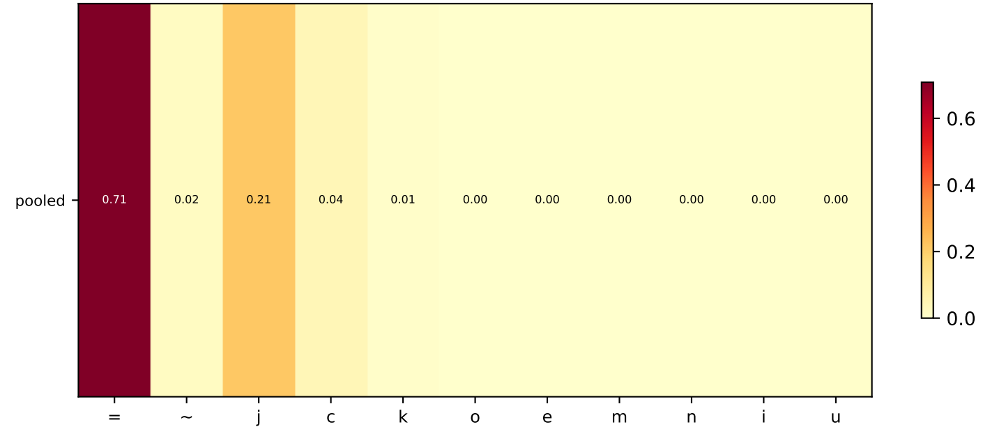
Fraction per species
