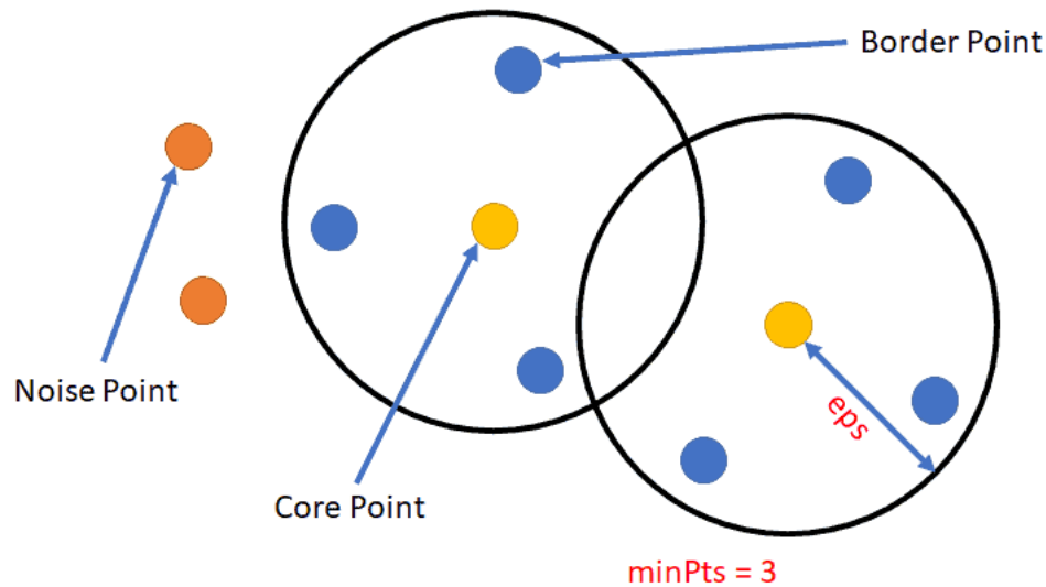
Abbildung 3.6.: Beispielhafte Darstellung von DB-Scan Algorithmus 2
