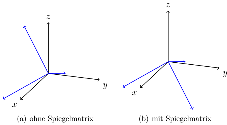
Abbildung 4.7.: Veränderung der Rotationmatrix durch die Spiegelmatrix
