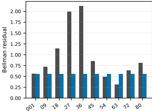
linear population
