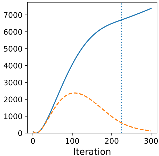
Homotopy: \tau = 1.0 \rightarrow 1e - 06
