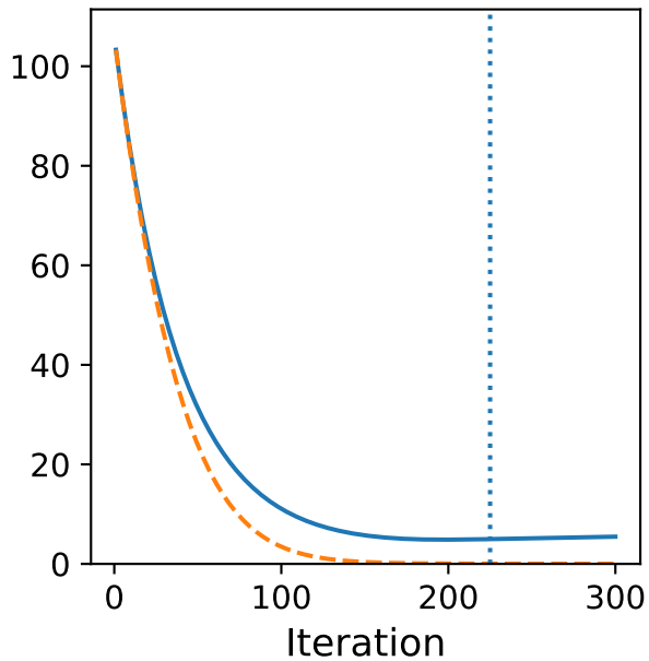
Homotopy: \tau = 0.1 \rightarrow 1e - 06
