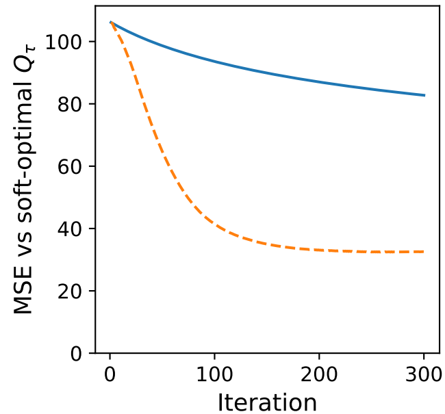
Fixed \tau = 1e - 06
