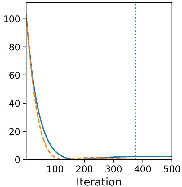
Homotopy: \tau = 0.1 \rightarrow 1e - 06
