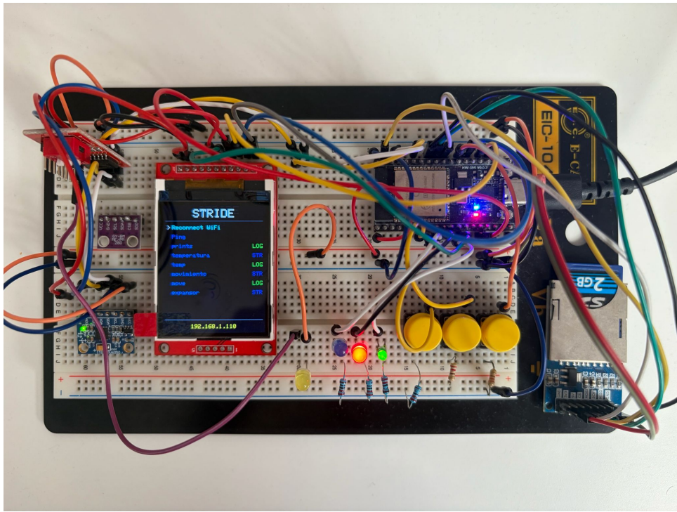
Figura 7.3: Dispositivo encendido mostrando la pantalla de inicio.
