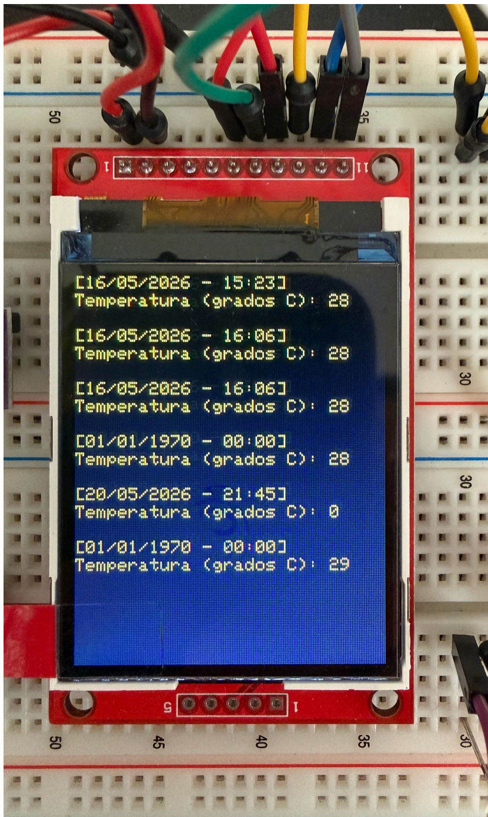
Figura 7.6: Registros ( logs ).
