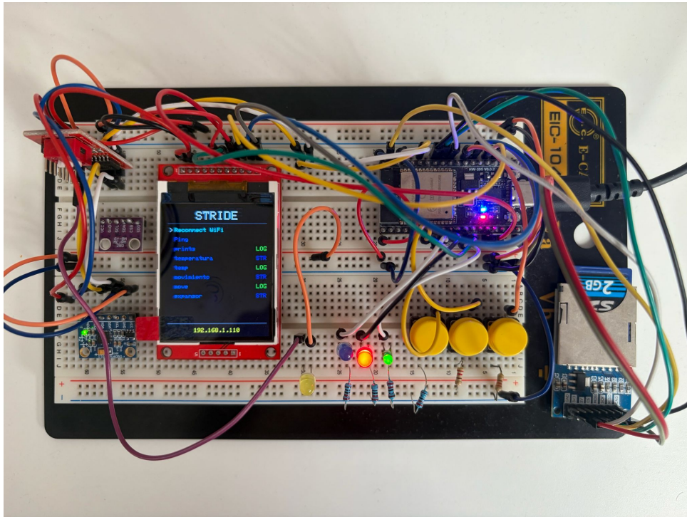
Figura 7.3: Dispositivo encendido.
