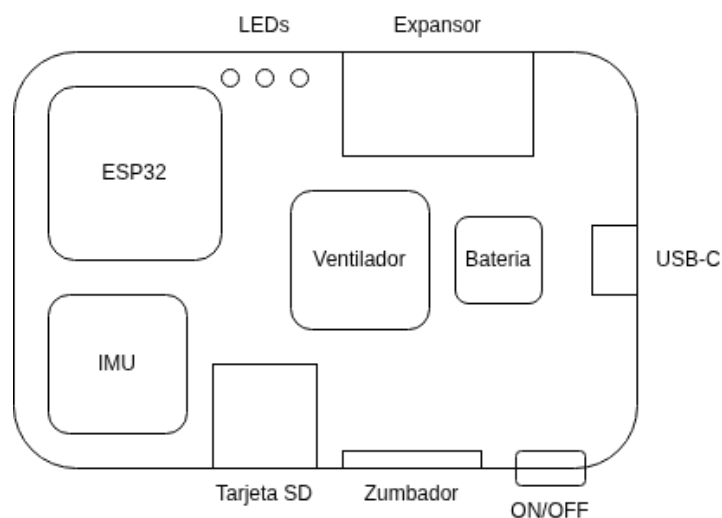
Figura 7.2: Distribución interna conceptual de los componentes.
