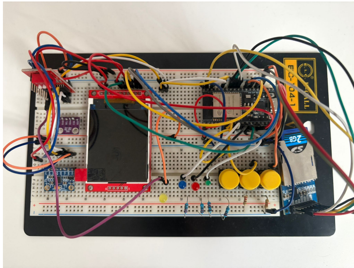
Figura 6.1: Prototipo del dispositivo desarrollado.
