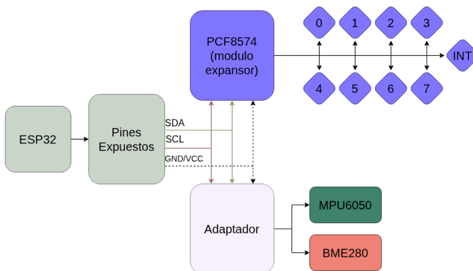
Figura 4.5: Representación conceptual de las conexiones.
