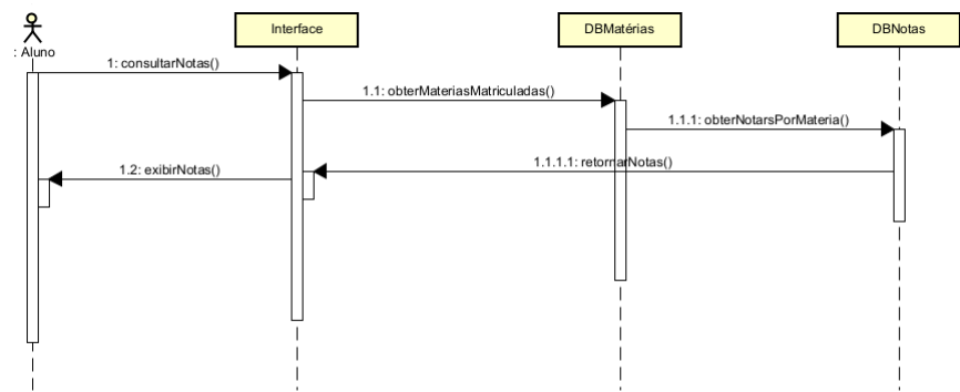
Figura 10 – Sequência: consulta de notas do aluno
