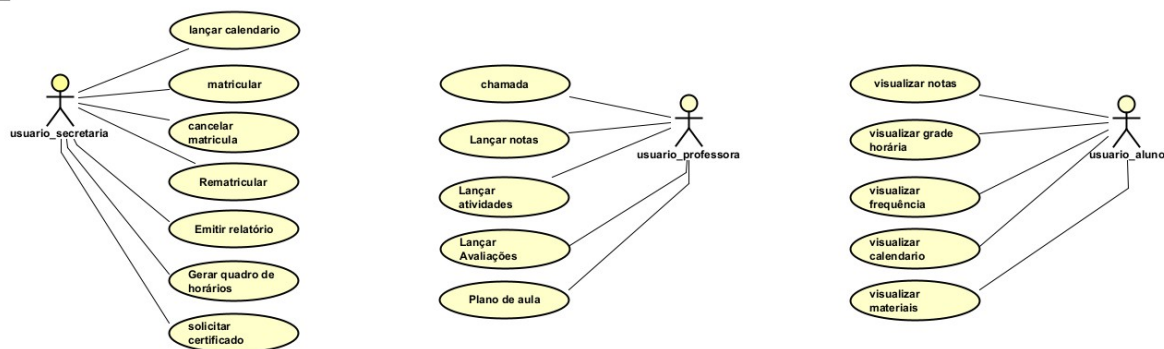
Figura 1 – Diagrama de casos de uso
