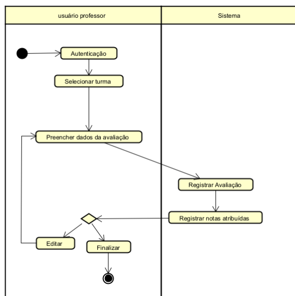
Figura 9 – Atividades: registro de notas dos alunos
