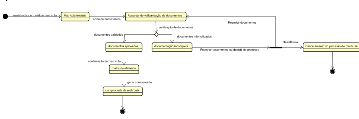
Figura 6 – Máquina de estados do processo de matrícula
