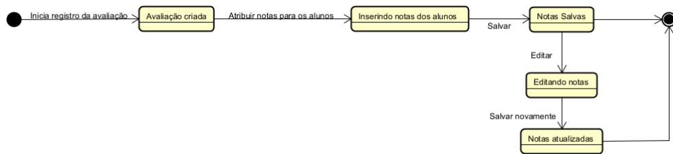
Figura 7 – Máquina de estados da criação de avaliação e inserção de notas
