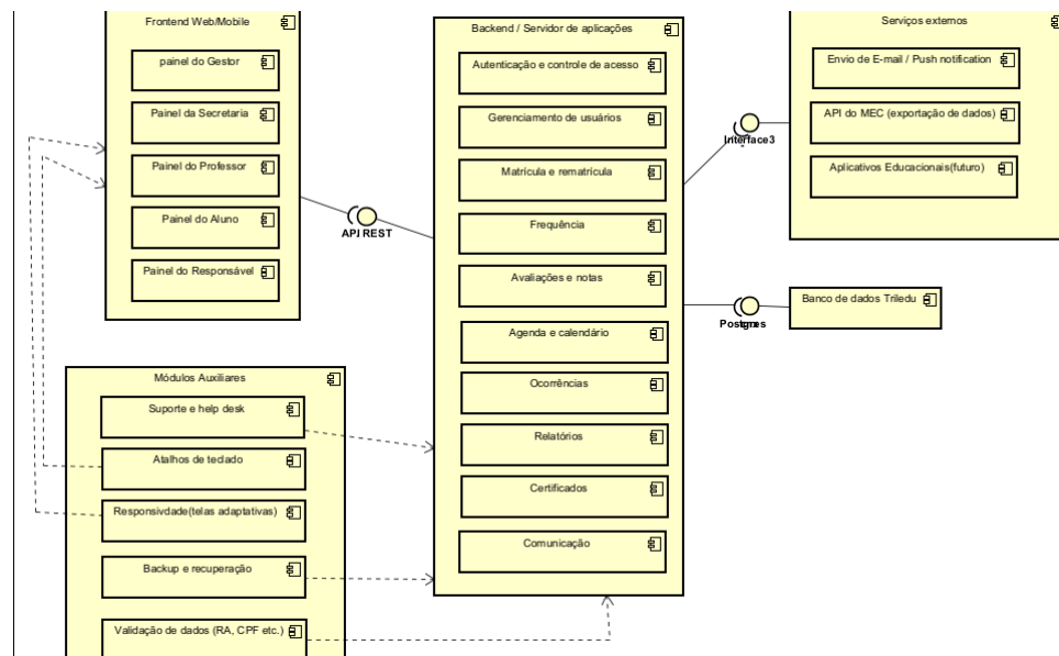
Figura 4 – Diagrama de componentes do sistema
