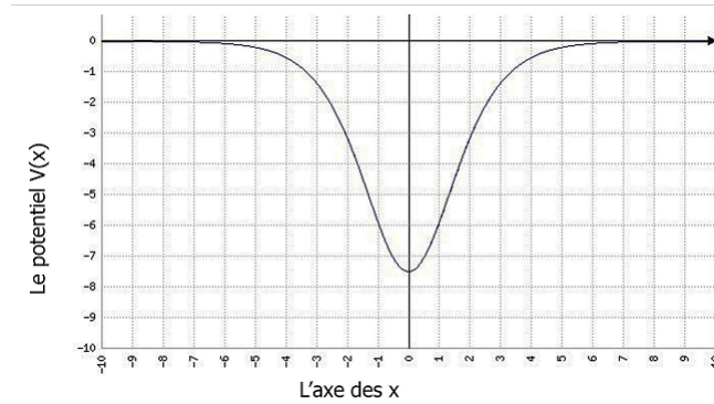
Figure 3.1 : Représentation graphique du potentiel de Pöschl-Teller pour A = -30 et \alpha = \frac{1}{2} .
