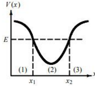
Figure 2.1 : Un mur de potentiel
