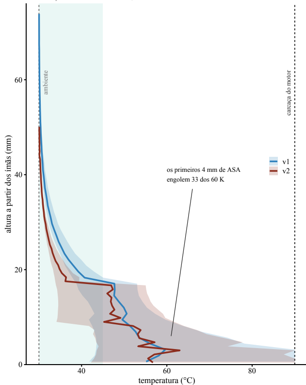
a Onde os 60 K se perdem faixa = espalhamento em cada cota; área clara = abaixo dos 45 °C da LiPo
