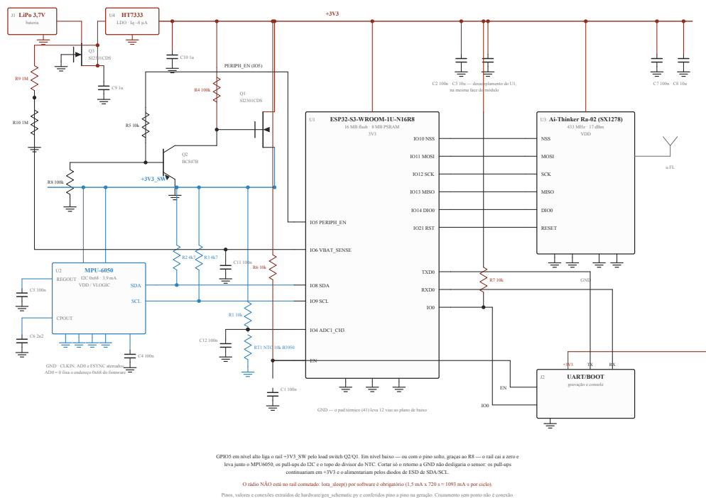
Figura 1 – Circuito de condicionamento e aquisição. Os valores da figura são gerados diretamente a partir das constantes do firmware, com o arquivo e a linha de origem registrados no cabeçalho do gerador.
