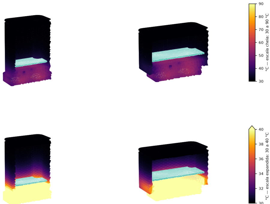
Figura 13 – Campo de temperatura em corte ( E ). A placa não integra o modelo de elementos finitos; sua temperatura provém de balanço radiativo calculado separadamente.
