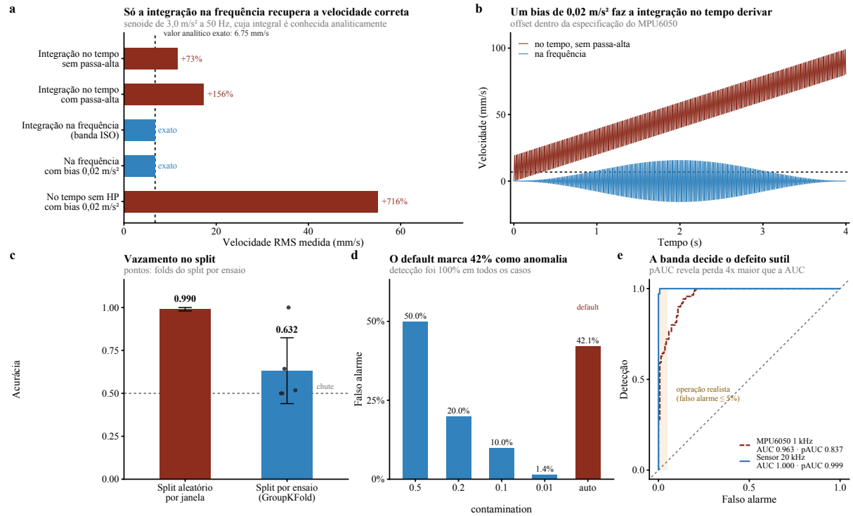
Figura 10 – Três escolhas metodológicas alteram os resultados mais do que o efeito medido (S). a , Velocidade eficaz por cinco variantes de integração contra o valor analítico exato; apenas a integração no domínio da frequência o recupera. b , Deriva causada por viés contido na especificação do sensor. c , Acurácia do mesmo modelo sobre os mesmos dados, variando apenas a estratégia de partição; pontos indicam as partições individuais. d , Fração da operação normal classificada como anomalia por valor do parâmetro de contaminação. e , Curvas ROC por banda de aquisição; a faixa sombreada marca a região de operação realista.
