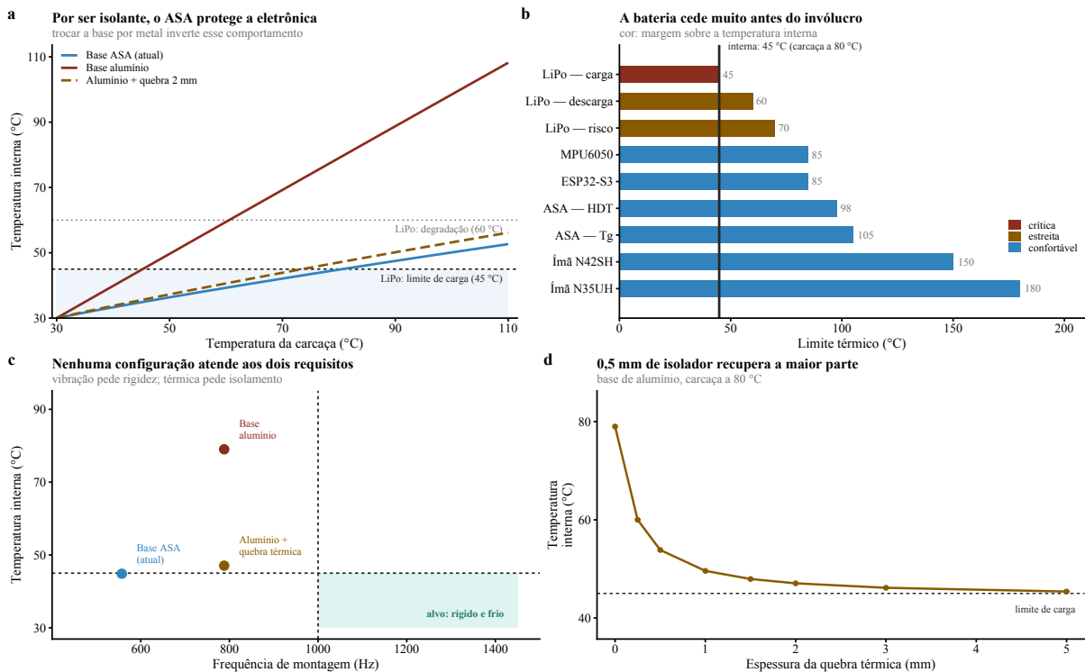
Figura 11 – A bateria, e não o invólucro, define a margem térmica ( ^{\text{E}} ). Por ser mau condutor, o polímero do invólucro mantém o interior em 44,8^{\circ}\text{C} com a carcaça a 80^{\circ}\text{C} ; o componente que atinge primeiro seu limite é a célula, pela restrição de carga em 45^{\circ}\text{C} .
