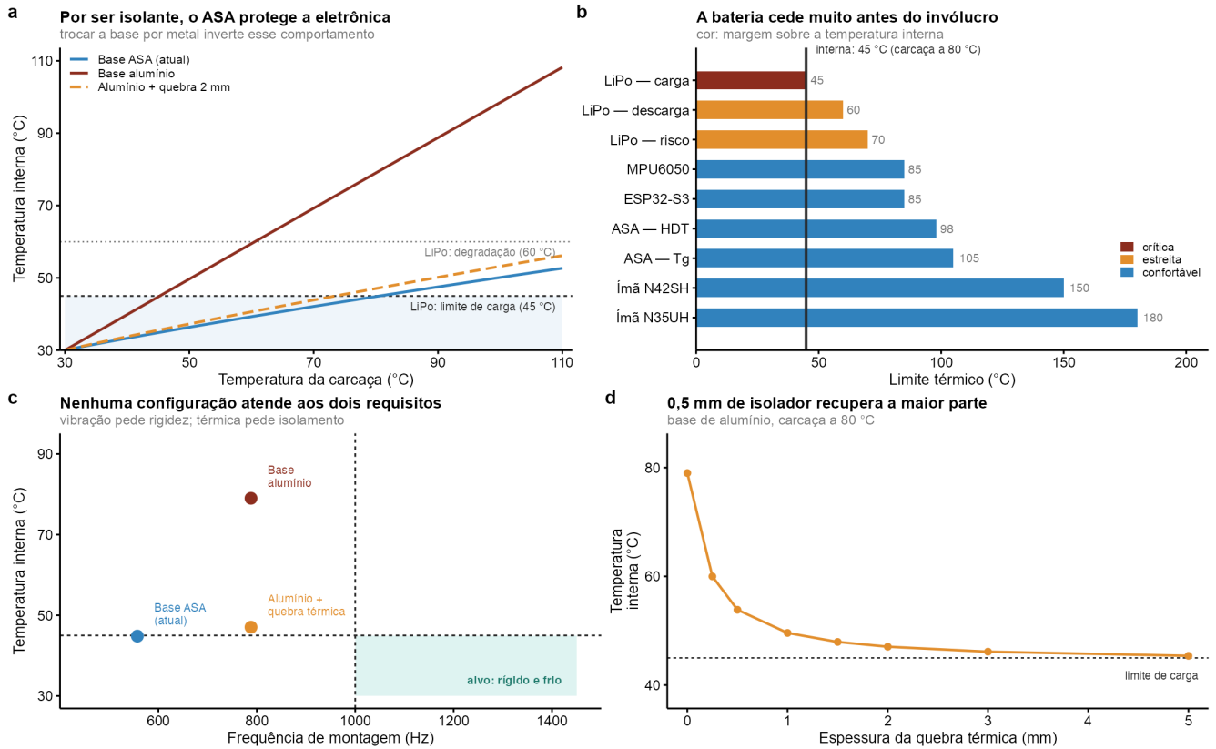
Figura 4: O ASA protege a eletrônica, e a bateria é o elo térmico mais fraco. a , Temperatura interna em regime permanente em função da temperatura da carça, para três configurações de base. b , Limite térmico de cada componente comparado à temperatura interna com carça a 80 °C; a cor indica a margem disponível. c , As duas análises impõem requisitos opostos à base, e nenhuma das três configurações alcança simultaneamente a região desejável. d , Temperatura interna com base metálica em função da espessura do espaçador isolante.
