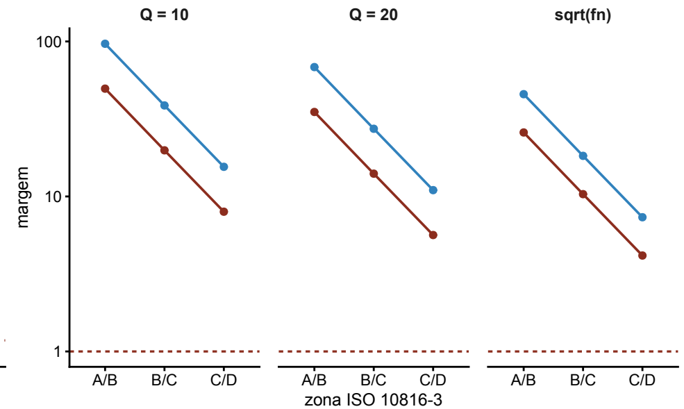
Figura 5: Transmissibilidade do caminho de montagem, margem de Steinberg por componente e sensibilidade ao amortecimento e à severidade.
